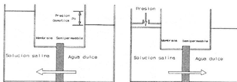
Figura 4a. Presión Osmótica
