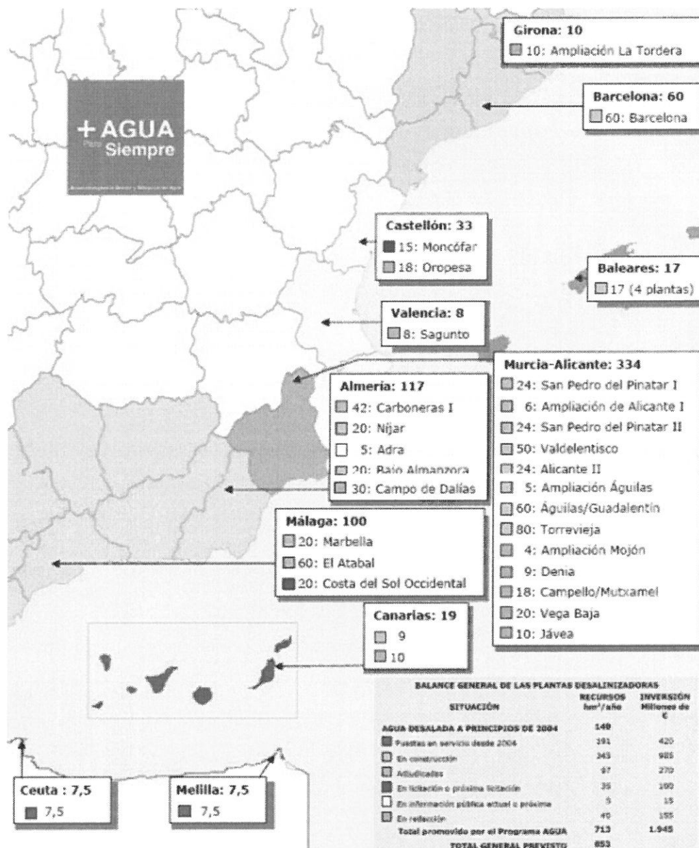
Mapa 3 - Situación de las plantas desalinizadoras del Programa A.G.U.A. (en hm 3 /año)
