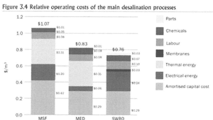
Gráfico 4 – Costes operativos relativos de los principales procesos de desalación
