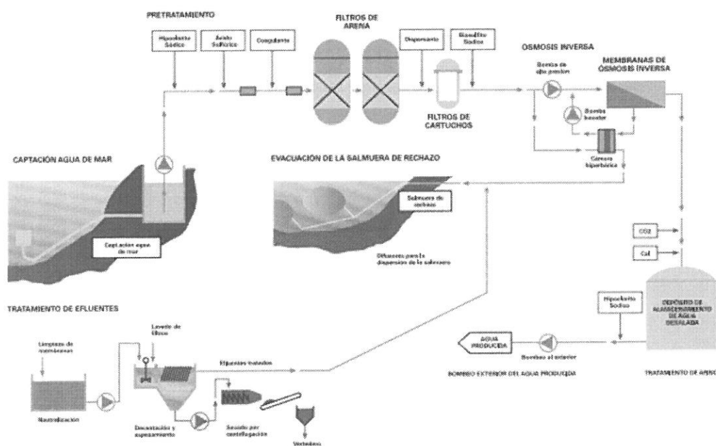
Gráfico 7 - Etapas de la ósmosis inversa
