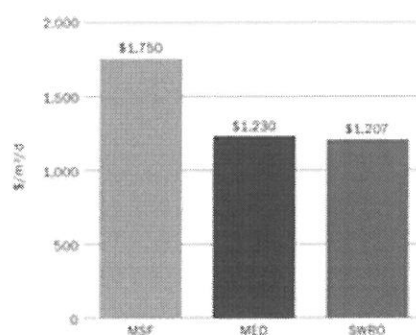
Gráfico 6 - Costes medios relativos EPC por m 3 de los principales procesos (grandes plantas)
