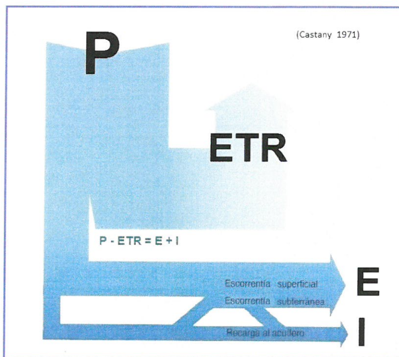
Figura 3. Esquema tomado del Libro Blanco del Agua (Ministerio de Medio Ambiente, 2001) y del Plan Hidrológico del Júcar 2009-2015 con las componenets del ciclo hídrico (Castany, 1971)
