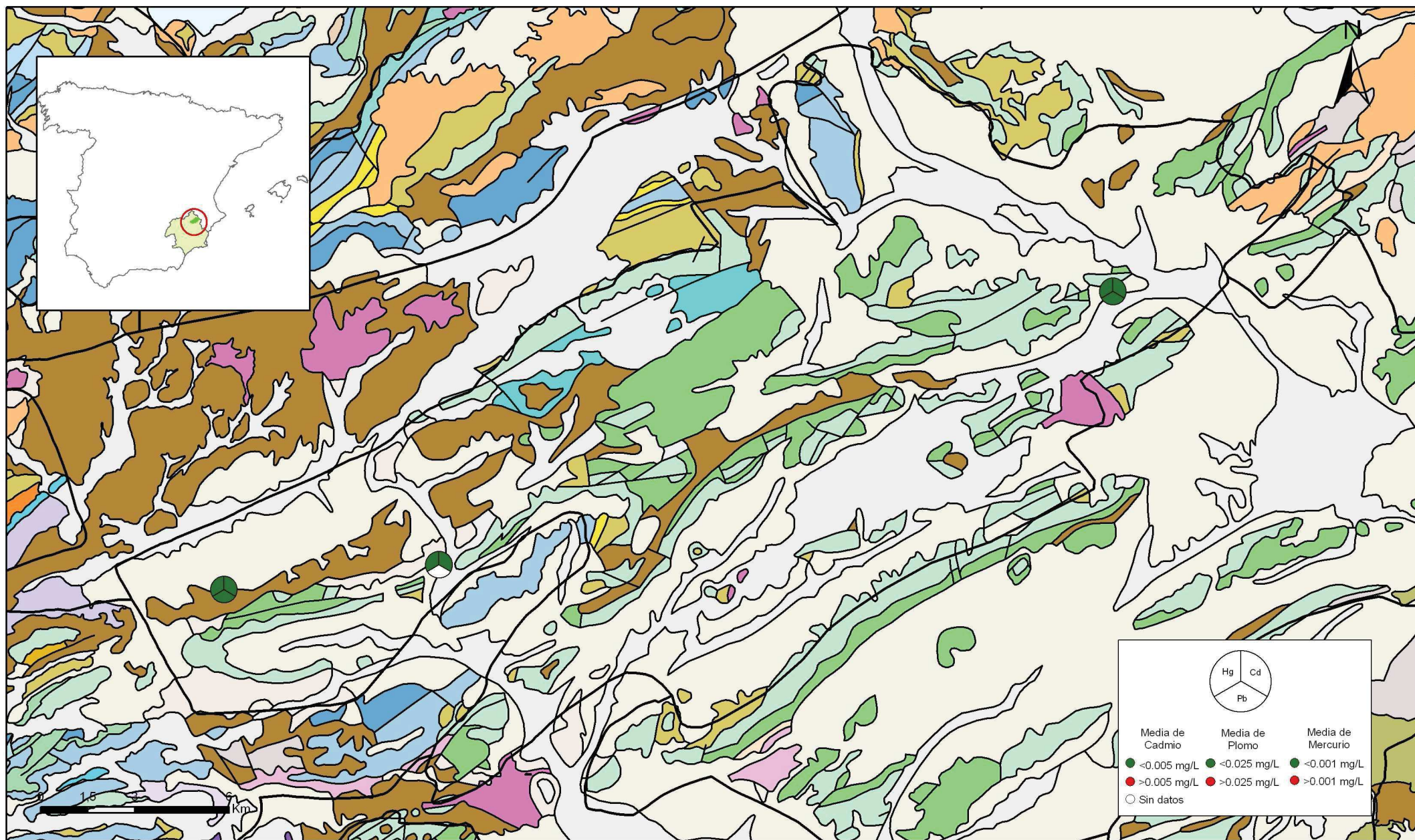
Mapa 10.3.3. Mapa de calidad química de referencia. Metales pesados de la masa Cingla (070.012)
