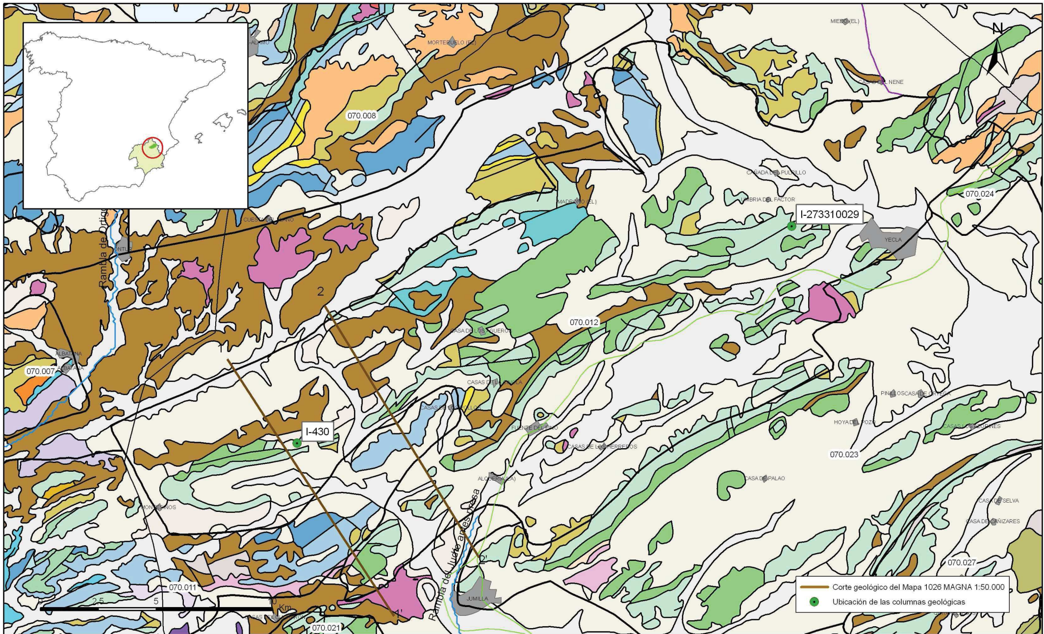
Mapa 2.1 Mapa geológico de la masa Cingla (070.012)
