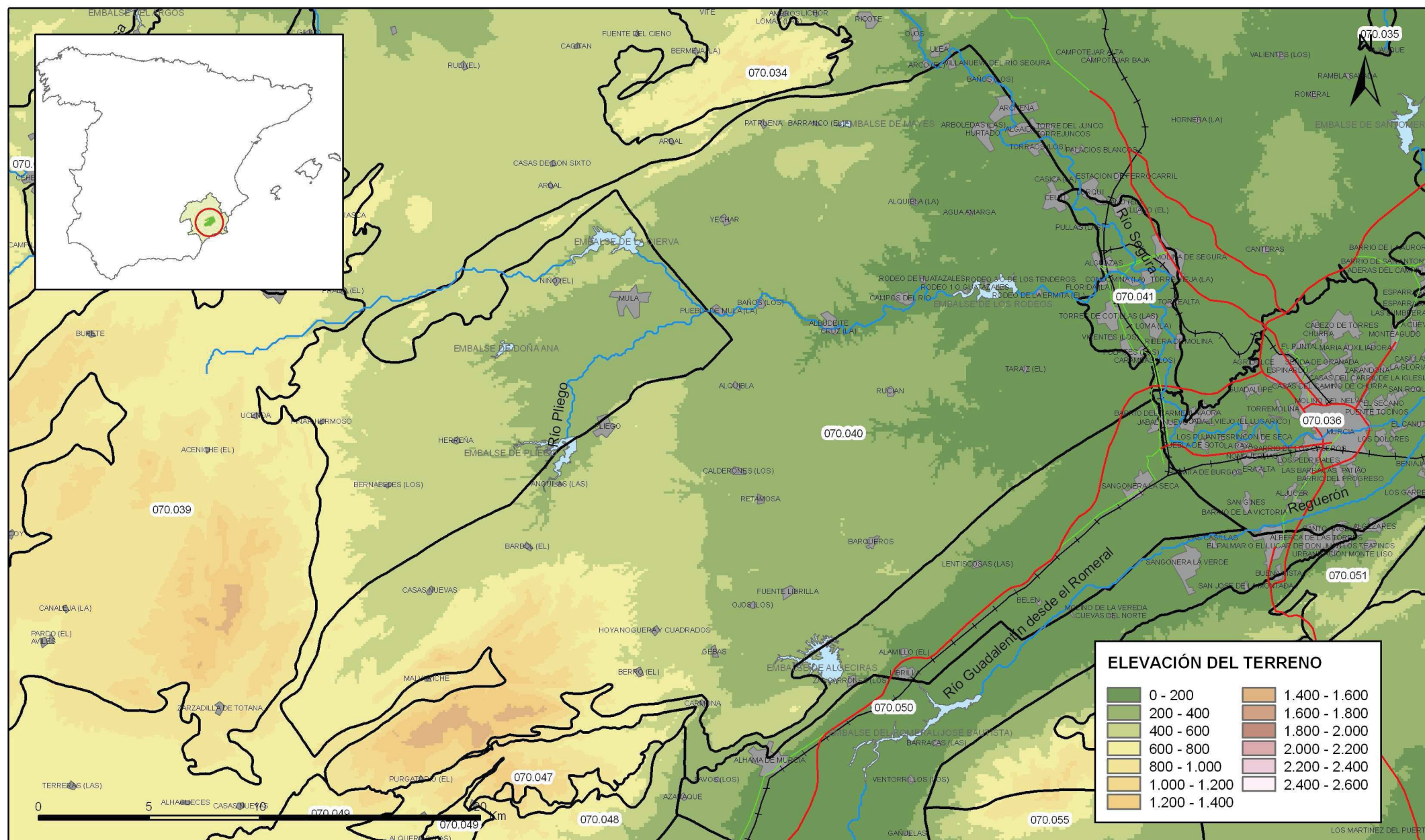
Mapa 1.2 Mapa digital de elevaciones de la masa Sierra Espuña (070.040)
