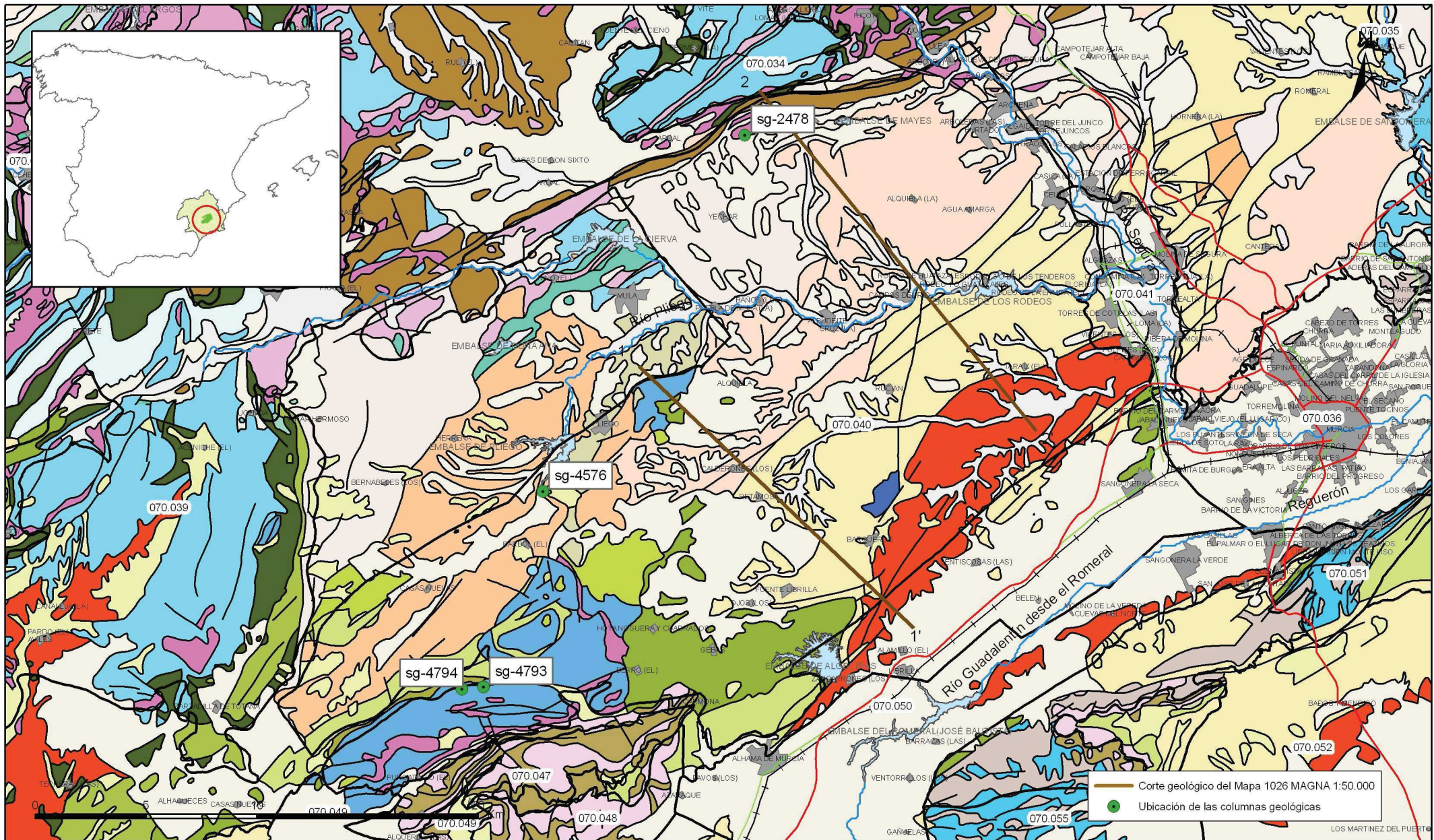
Mapa 2.1 Mapa geológico de la masa Sierra Espuña (070.040)
