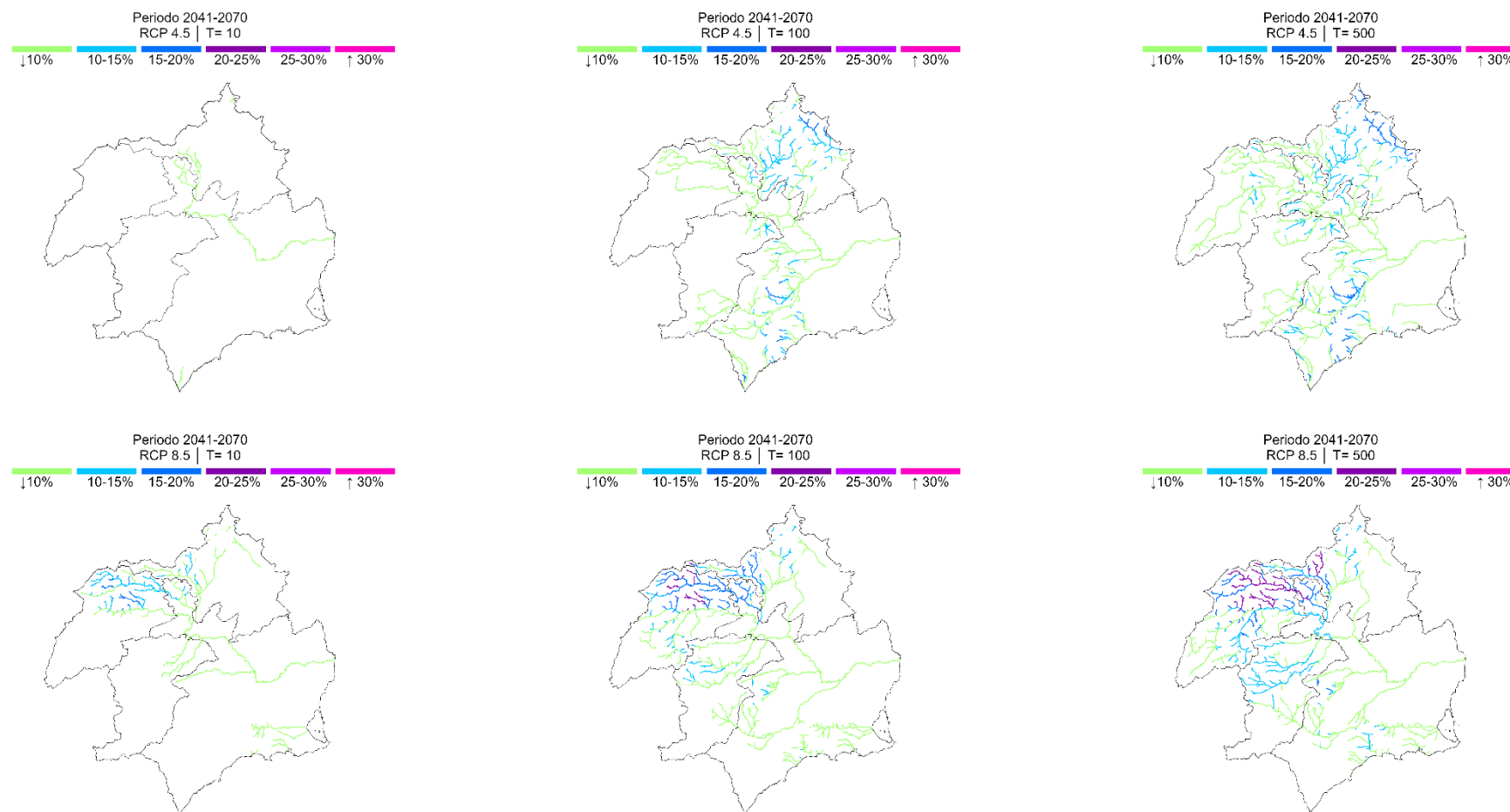
Figura 60. Tasa de cambio de la precipitación máxima acumulada en la red fluvial proyectada bajo los escenarios medio (RCP 4.5) y pesimista (RCP 8.5) de emisiones para el horizonte temporal 2041-2070, y para los periodos de retorno de 10, 100 y 500 años, calculada respecto al periodo de control (1971-2000). Fuente: Elaboración propia a partir de información del CEDEX
