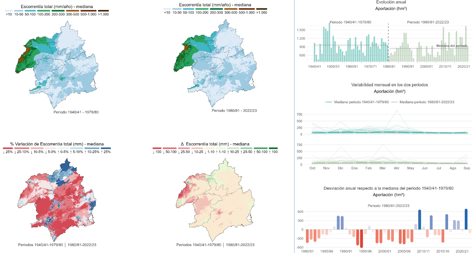
Figura 32. Caracterización espacial y temporal de la aportación. Comparación entre los periodos 1940/41–1979/80 y 1980/81–2022/23. Fuente: Elaboración propia a partir de información de SIMPA (CEDEX).
