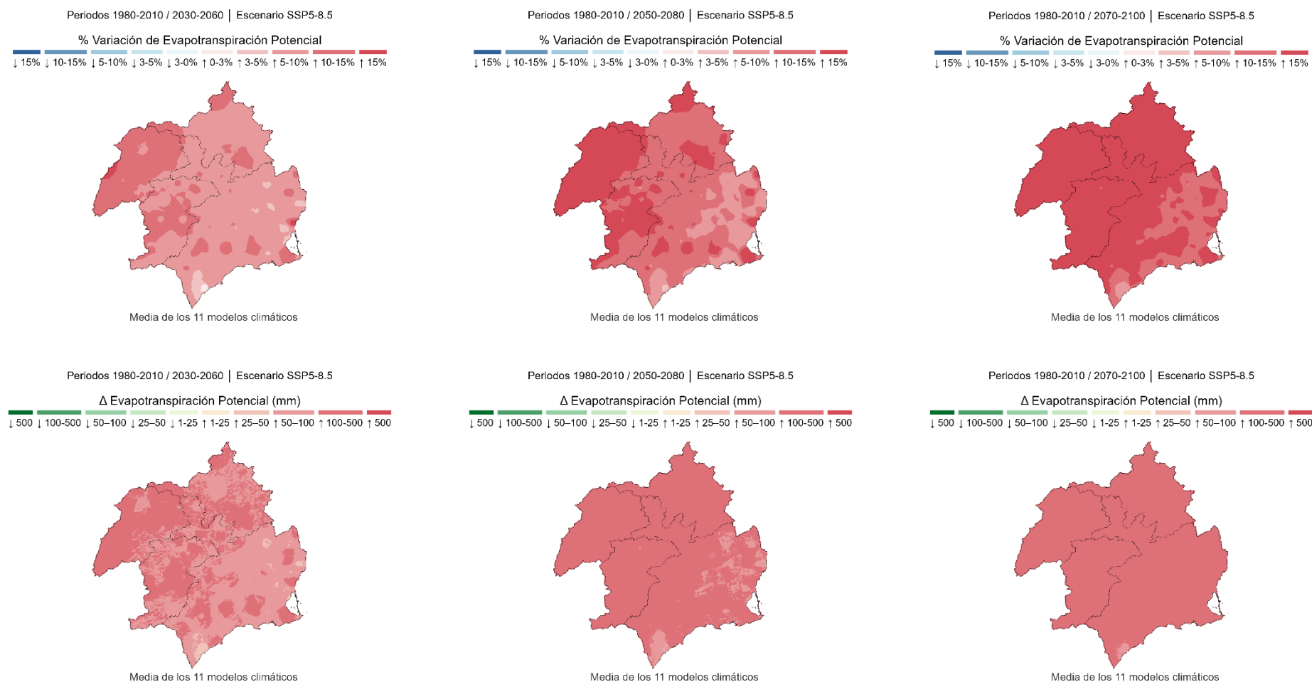
Figura 51. Variación de la evapotranspiración potencial proyectada bajo el escenario pesimista de emisiones (SSP5-8.5), para los horizontes temporales 2030-2060, 2050-2080 Y 2070-2100, en comparación con el periodo de control 1980-2010. Fuente: Elaboración propia a partir de información del CEDEX, 2025.
