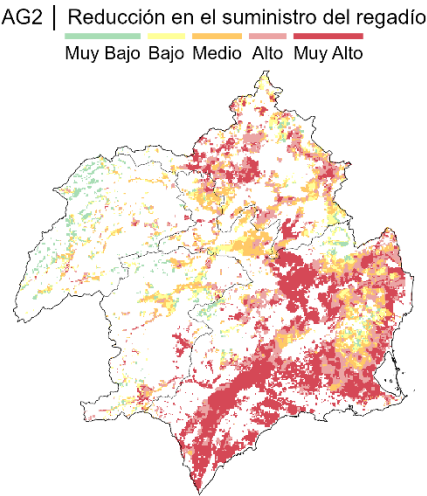
Figura 127. Riesgo AG2: Mapa de situación actual (periodo 1980/81 – 2022/23)
