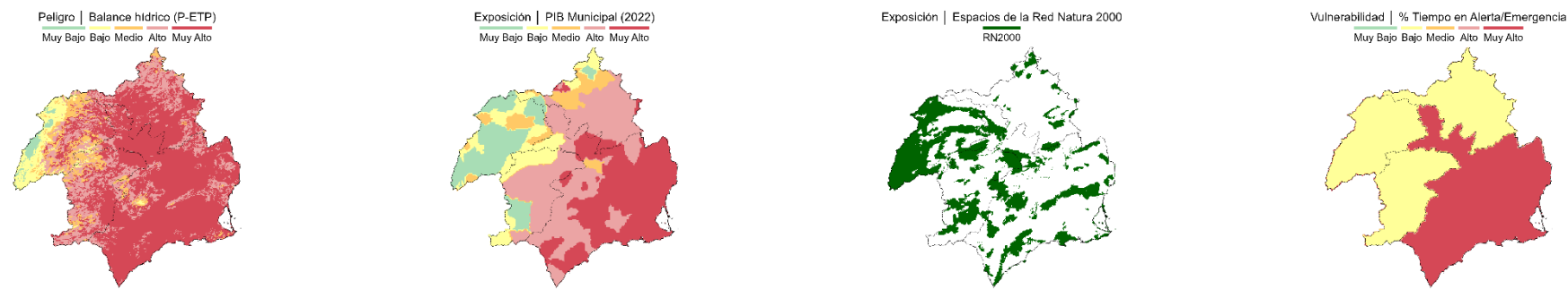
Figura 105. Riesgo ECS9. Mapas de los indicadores de peligro, exposición y vulnerabilidad
