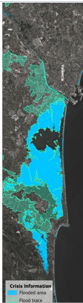
Extensión de las inundaciones de octubre de 2024 en el entorno de un humedal del Mediterráneo. (octubre de 2024), Fuente: Copernicus (Unión Europea)
