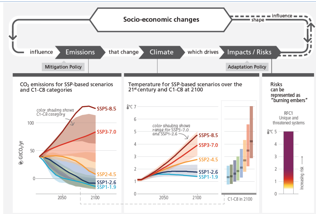
Figura 37. Representación de la cadena causa-efecto embebida en los SSP. Fuente: AR6
