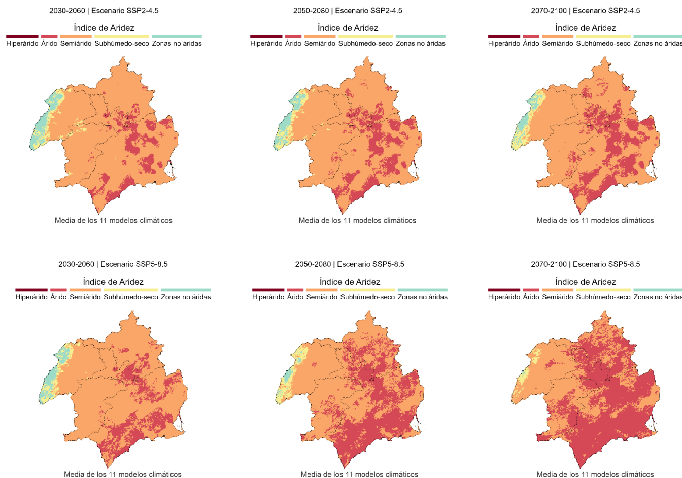
Figura 65. Variación del índice de aridez para diversos horizontes temporales y escenarios climáticos. Fuente: elaboración propia a partir de proyecciones SIMPA (CEDEX)
