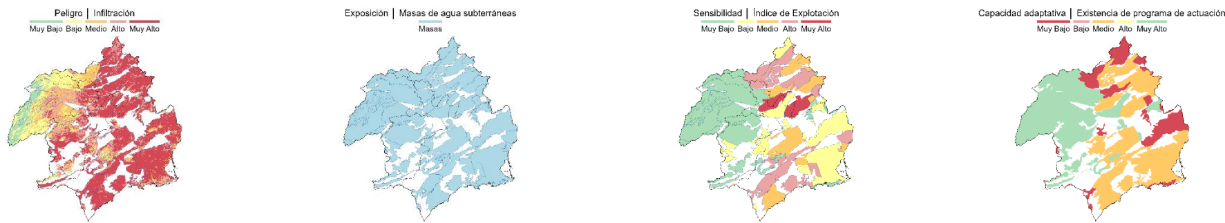
Figura 87. Riesgo GW3. Mapas de los indicadores de peligro, exposición y vulnerabilidad (sensibilidad y capacidad adaptativa)
