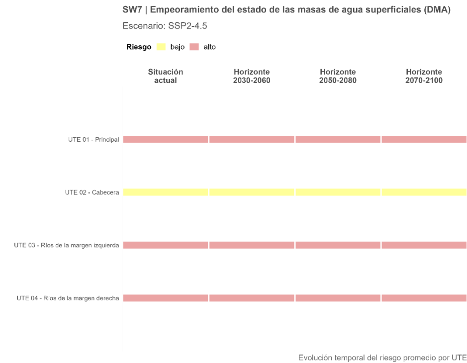
Figura 85. Trayectoria temporal del riesgo SW7 promedio por UTE, proyectado bajo el escenario intermedio (SSP2-4.5).
