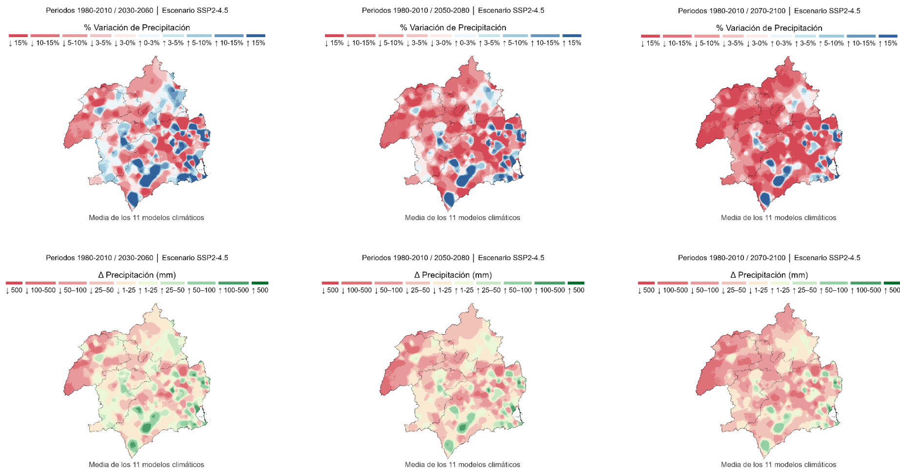
Figura 48. Variación de la precipitación proyectada bajo el escenario intermedio de emisiones (SSP2-4.5), para los horizontes temporales 2030-2060, 2050-2080 Y 2070-2100, en comparación con el periodo de control 1980-2010. Fuente: Elaboración propia a partir de información del CEDEX, 2025.
