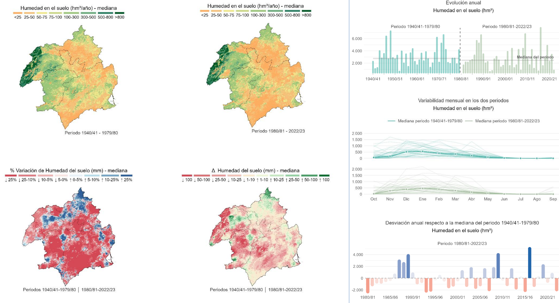
Figura 26. Caracterización espacial y temporal de la humedad en el suelo. Comparación entre los periodos 1940/41–1979/80 y 1980/81–2022/23. Fuente: Elaboración propia a partir de información de SIMPA (CEDEX).
