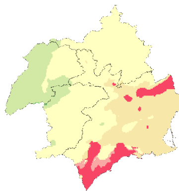
Clasificación climática de Köppen-Geiger (2011-2040) | Escenario SSP5-8.5
