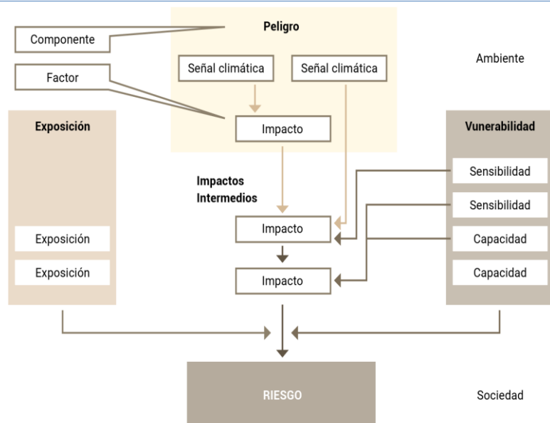
Figura 72. Esquema de componentes de los riesgos asociados al cambio climático (OECC 2023), adaptado de Risk Supplement to the Vulnerability Sourcebook (GIZ, 2017)
