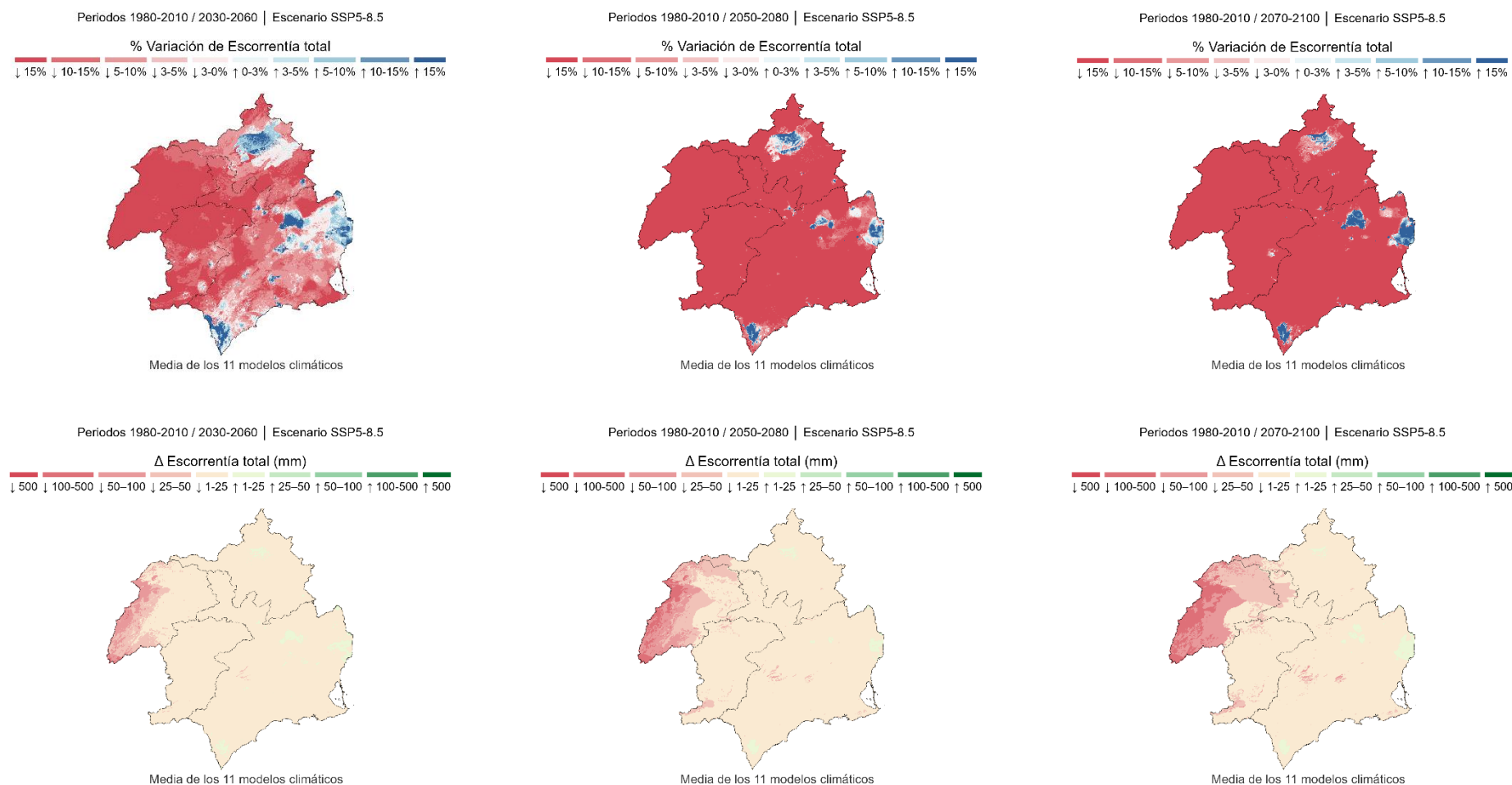
Figura 57. Variación de las aportaciones totales proyectadas bajo el escenario de altas emisiones (SSP5-8.5), para los horizontes temporales 2030-2060, 2050-2080 Y 2070-2100, en comparación con el periodo de control 1980-2010. Fuente: Elaboración propia a partir de información del CEDEX, 2025.
