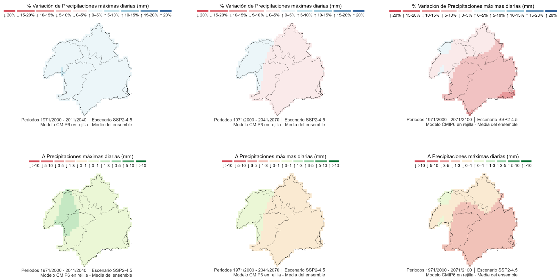
Figura 61. Variación de las precipitaciones máximas diarias proyectadas bajo el escenario intermedio de emisiones (SSP2-4.5), para los horizontes temporales 2011-2040, 2041-2070 y 2071-2100, en comparación con el periodo de control 1971-2000. Fuente: elaboración propia a partir de información de AdaptecCa
