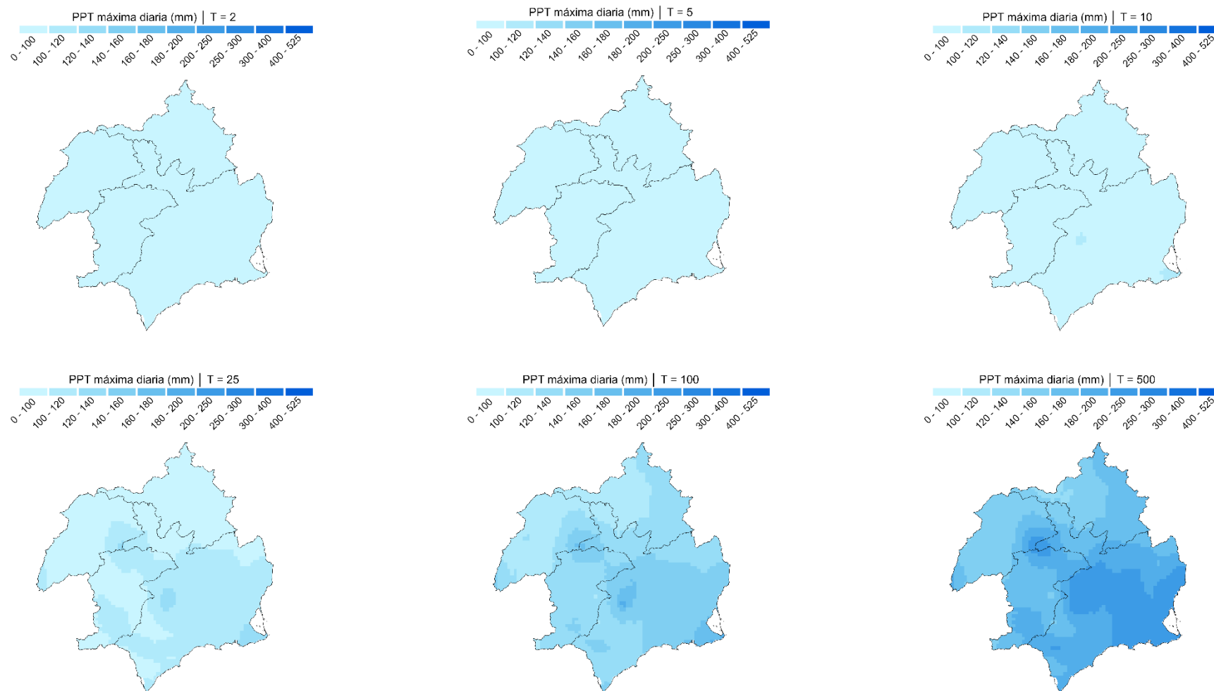
Figura 34. Caracterización espacial de las precipitaciones máximas diarias para los periodos de retorno de 2, 5, 10, 25, 100 y 500 años. Fuente: CAUMAX, 2014.
