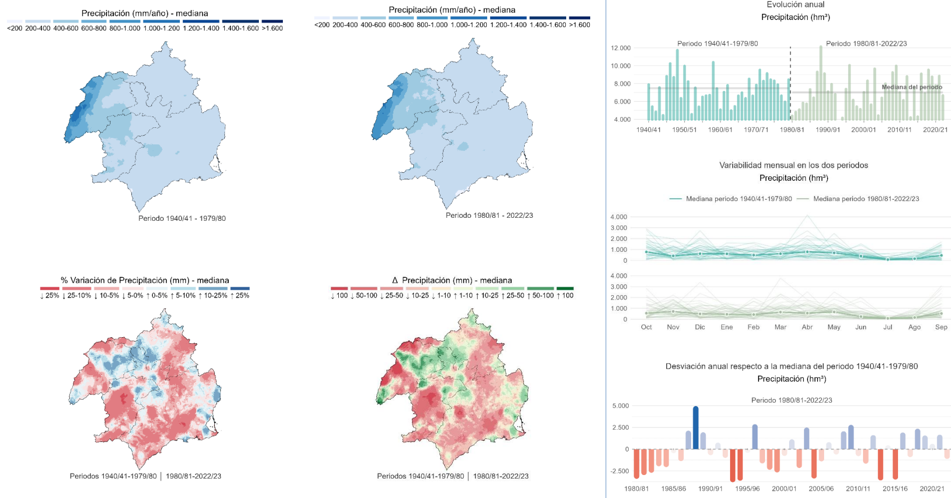
Figura 24. Caracterización espacial y temporal de la precipitación. Comparación entre los periodos 1940/41–1979/80 y 1980/81–2022/23. Fuente: Elaboración propia a partir de información de SIMPA (CEDEX).
