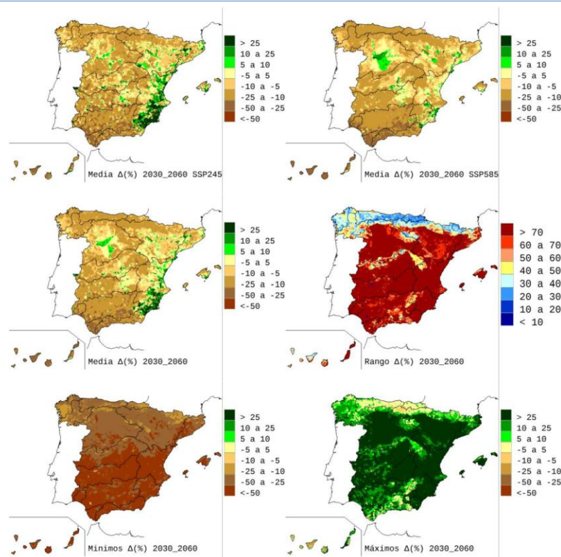
Figura 38. \Delta (%) ESC anual para 2030-2060 según el conjunto de las proyecciones. Arriba: media para cada SSP; medio: media y rango para ambos SSP; abajo: valores mínimos y máximos de cambio para ambos SSP. Fuente: «Nota técnica sobre la propuesta de incorporación del cambio climático en los planes hidrológicos del cuarto ciclo» (CEDEX 2025)
