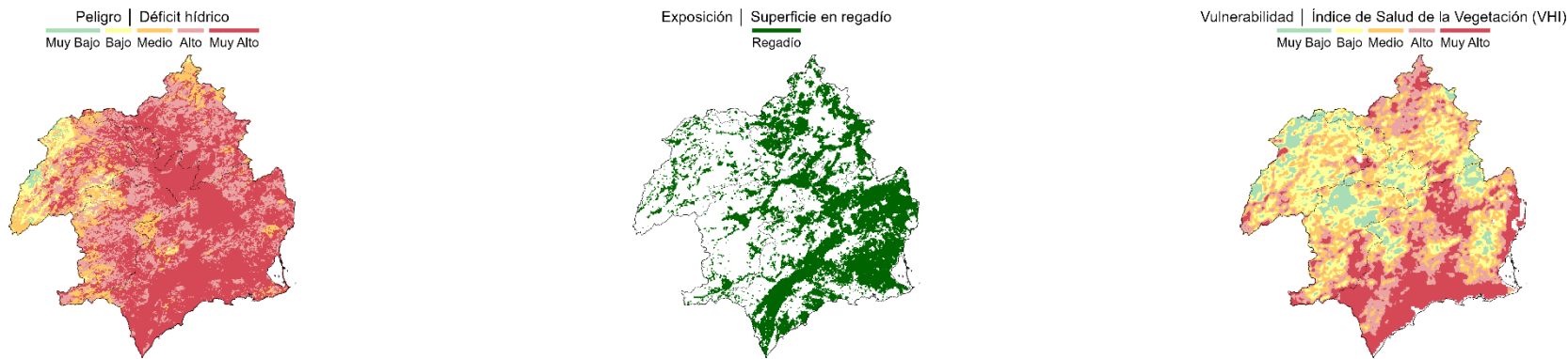
Figura 126. Riesgo AG2. Mapas de los indicadores de peligro, exposición y vulnerabilidad
