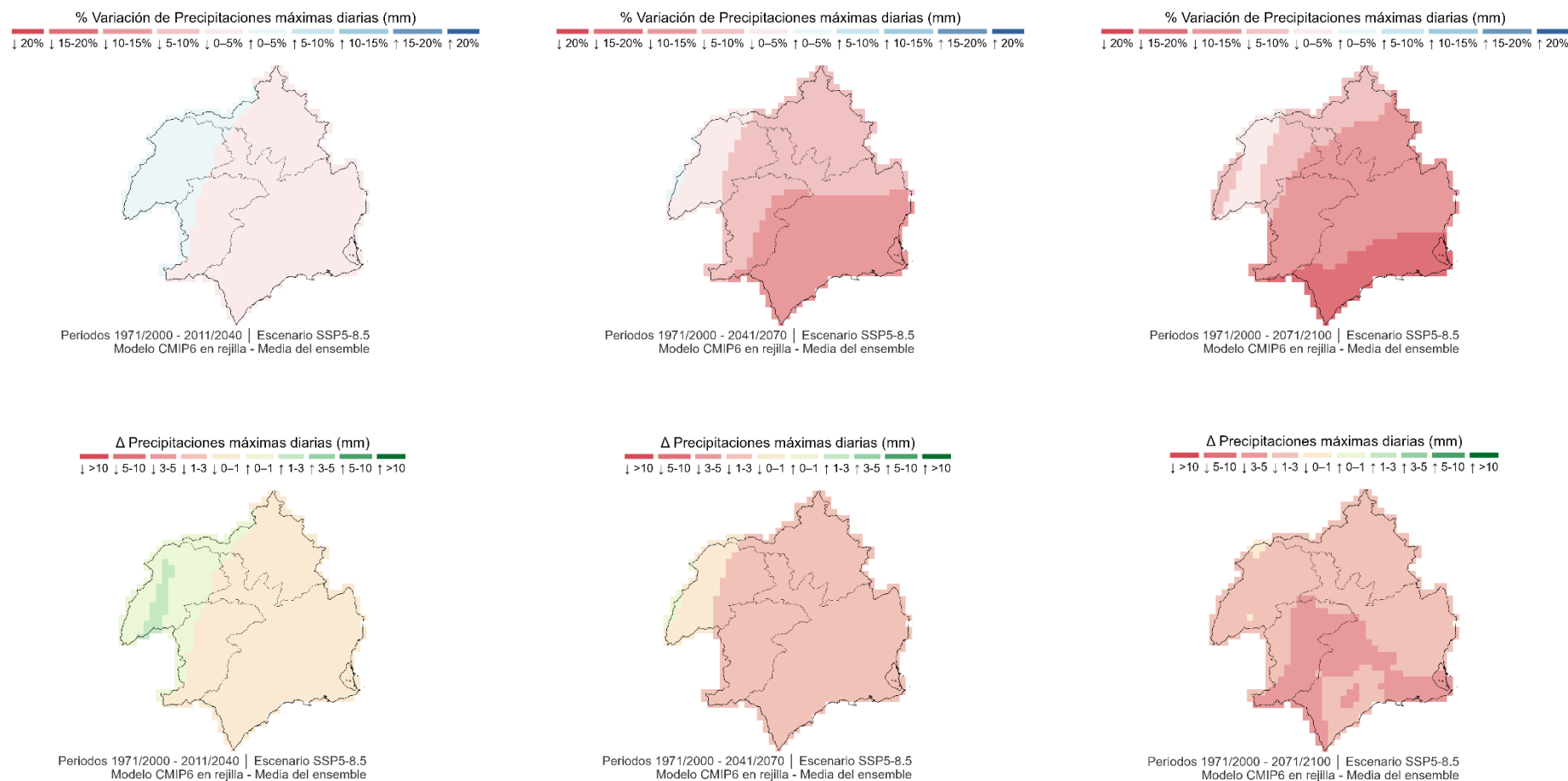
Figura 62. Variación de las precipitaciones máximas diarias proyectadas bajo el escenario de altas emisiones (SSP5-8.5), para los horizontes temporales 2011-2040, 2041-2070 y 2071-2100, en comparación con el periodo de control 1971-2000. Fuente: Elaboración propia a partir de información de AdaptecCa.
