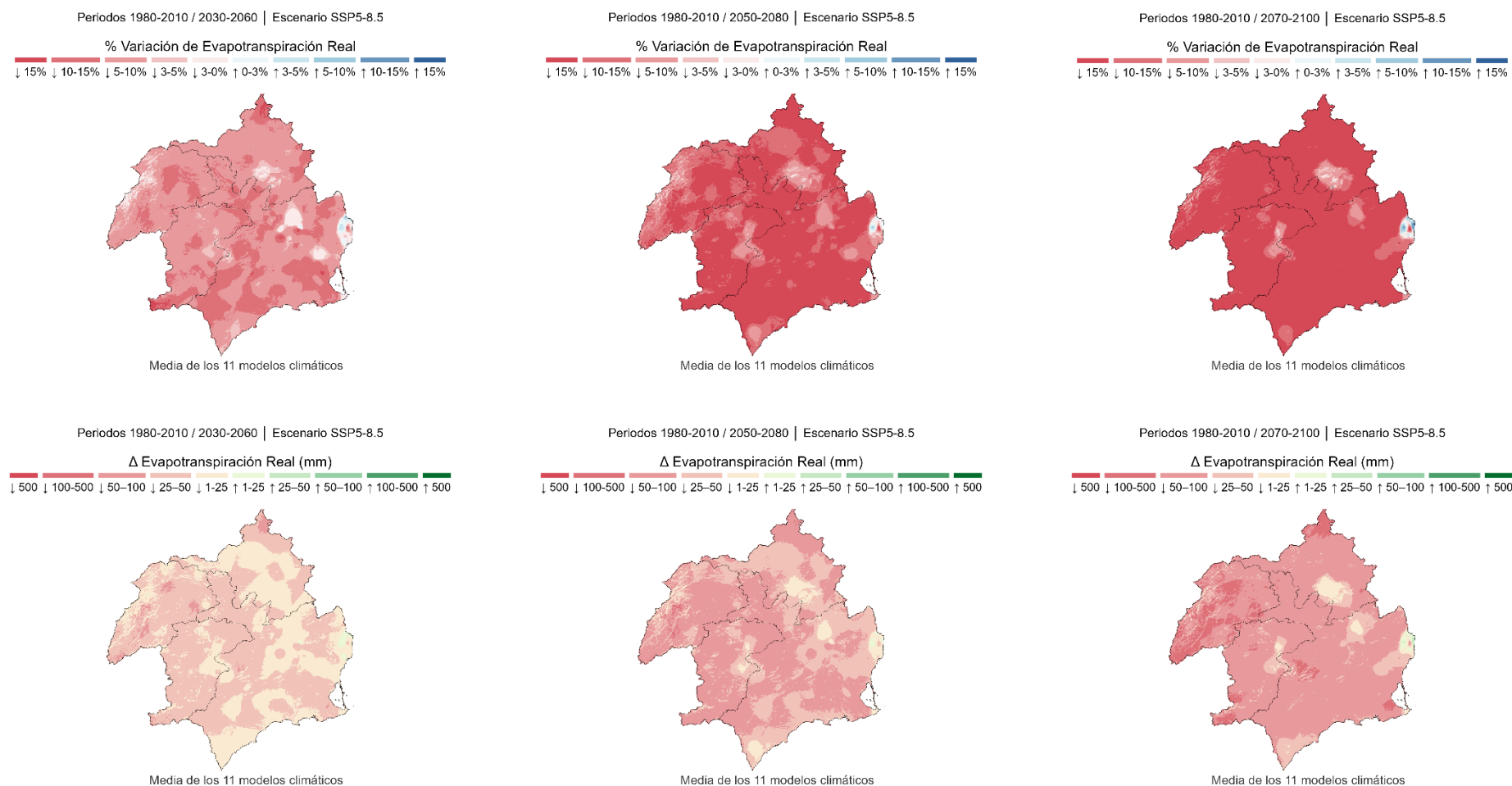
Figura 55. Variación de la evapotranspiración real proyectada bajo el escenario de altas emisiones (SSP5-8.5), para los horizontes temporales 2030-2060, 2050-2080 Y 2070-2100, en comparación con el periodo de control 1980-2010. Fuente: Elaboración propia a partir de información del CEDEX, 2025.
