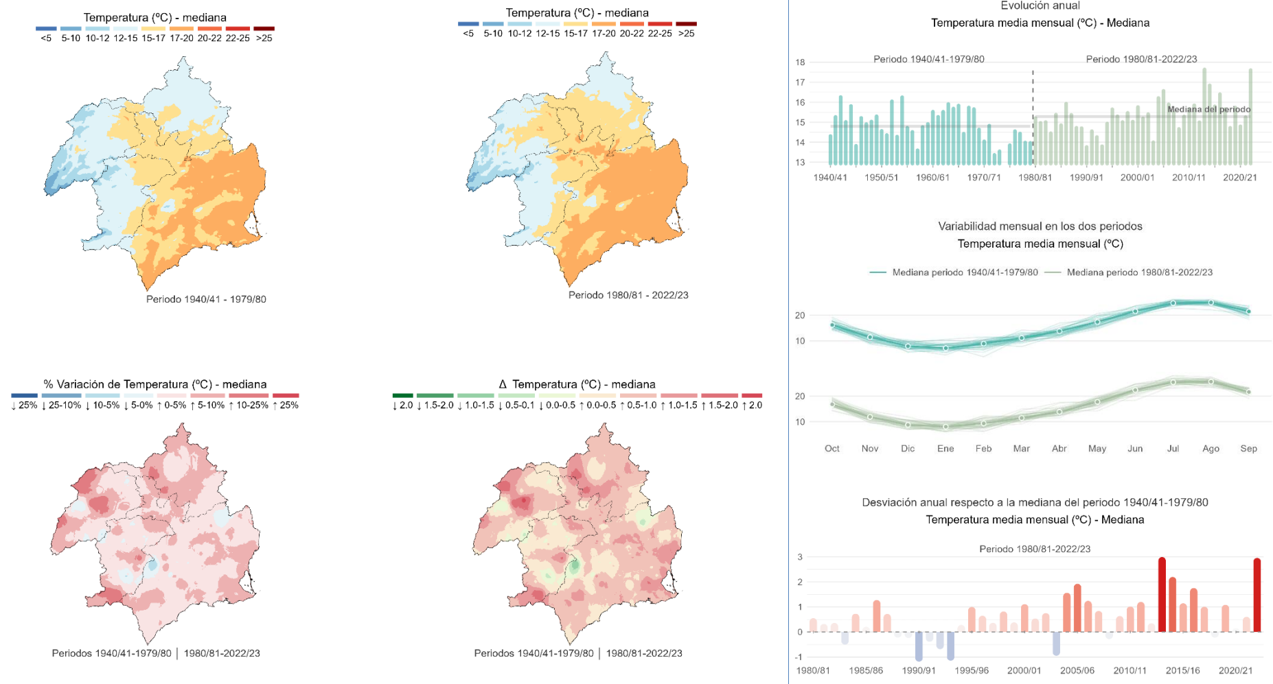
Figura 21. Caracterización espacial y temporal de la temperatura mediana. Comparación entre los periodos 1940/41–1979/80 y 1980/81–2022/23. Fuente: Elaboración propia a partir de información de SIMPA (CEDEX).
