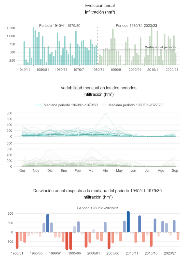
Figura 27. Caracterización espacial y temporal de la infiltración. Comparación entre los periodos 1940/41–1979/80 y 1980/81–2022/23. Fuente: Elaboración propia a partir de información de SIMPA (CEDEX).
