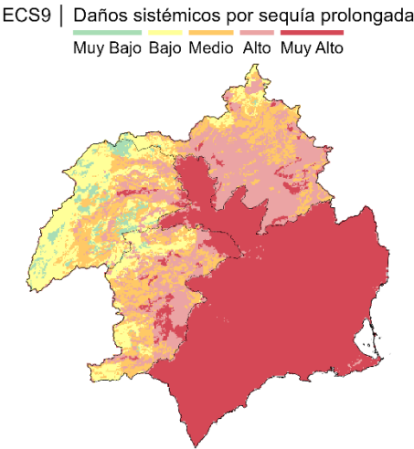
Figura 106. Riesgo ECS9: Mapa de situación actual (periodo 1980/81 – 2022/23)
