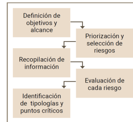
Figura 71. Esquema para la evaluación de los riesgos climáticos. Fuente OECC 2023
