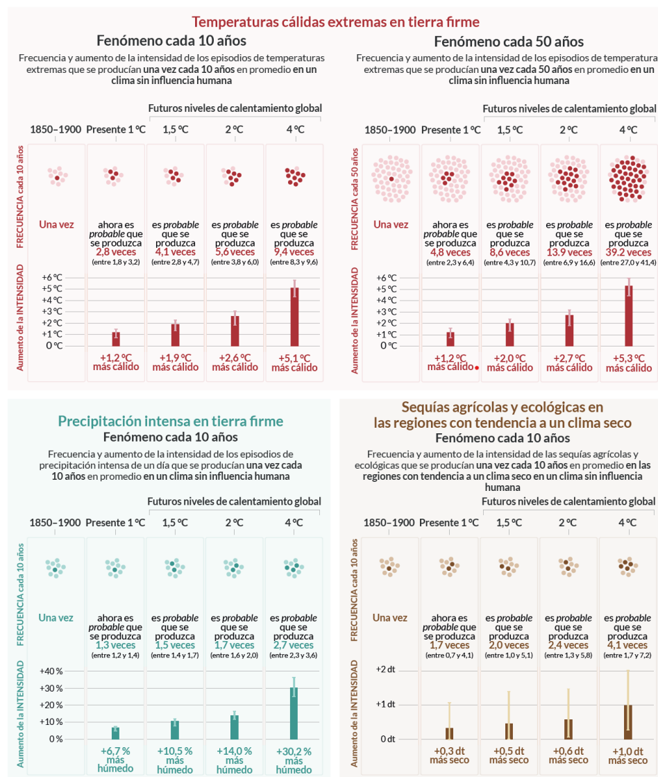
Figura 43. Evolución de los fenómenos extremos en intensidad y frecuencia
