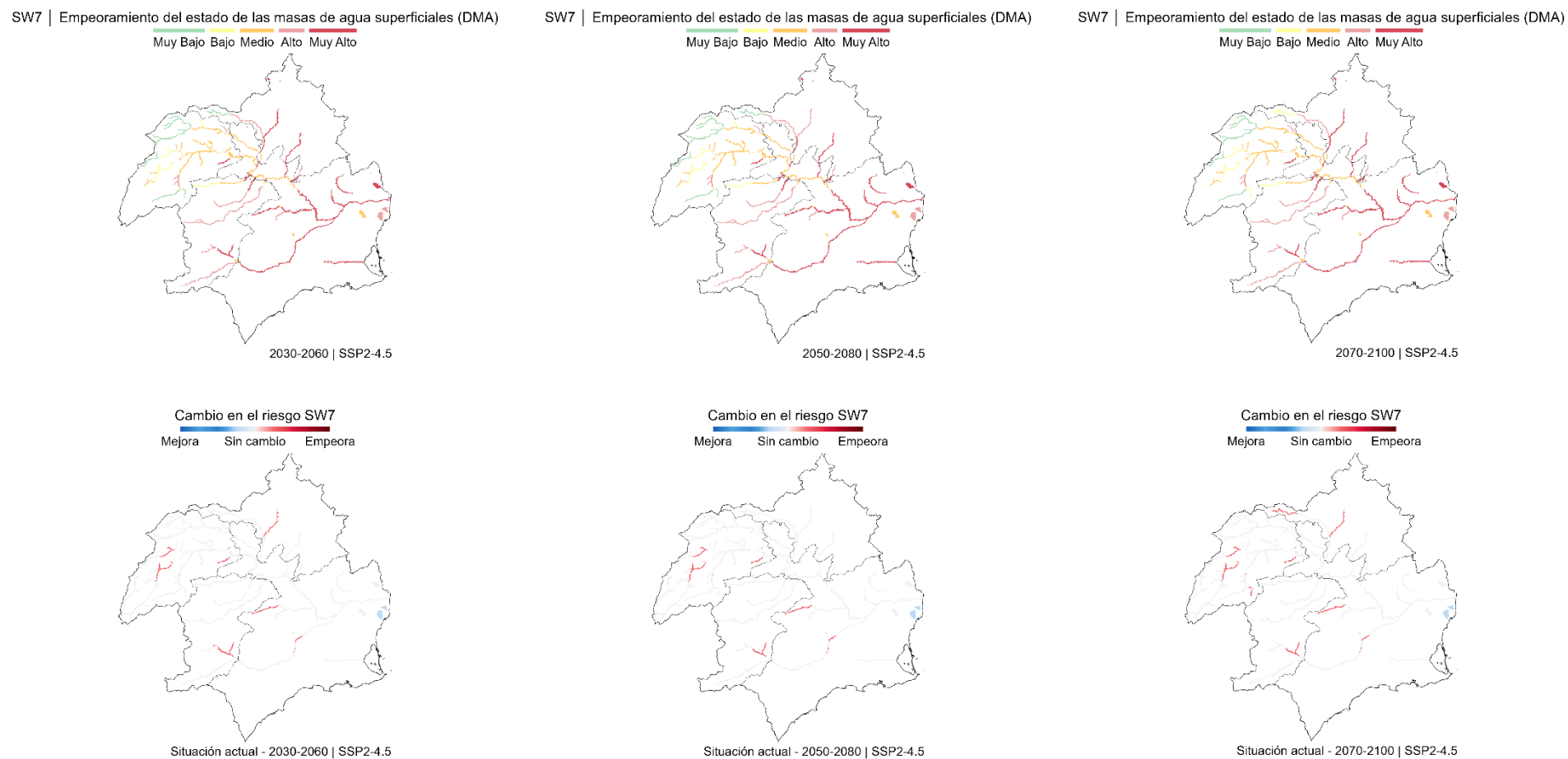
Figura 83. Evaluación del riesgo SW7 proyectado bajo el escenario intermedio (SSP2-4.5), para los horizontes temporales 2030-2060, 2050-2080 y 2070-2100 respecto a la situación de riesgo actual.
