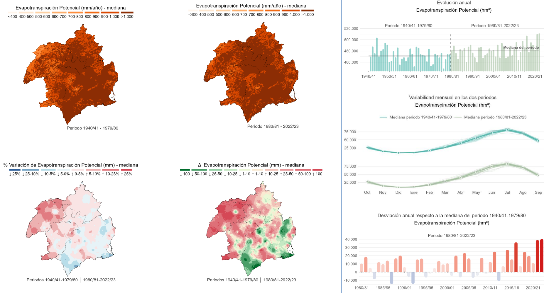
Figura 23. Caracterización espacial y temporal de la evapotranspiración potencial. Comparación entre los periodos 1940/41–1979/80 y 1980/81–2022/23. Fuente: Elaboración propia a partir de información de SIMPA (CEDEX). La mediana del periodo 1980/81–2022/23 (21.076,65 hm 3 ) supera a la del periodo 1940/41–1979/80 (20.632,55 hm 3 ) en 444,10 hm 3 , lo que supone un incremento del 2,15 %. La mayor desviación se produce en el año hidrológico 2022/23, siendo esta de +1.671,54 hm 3 .
