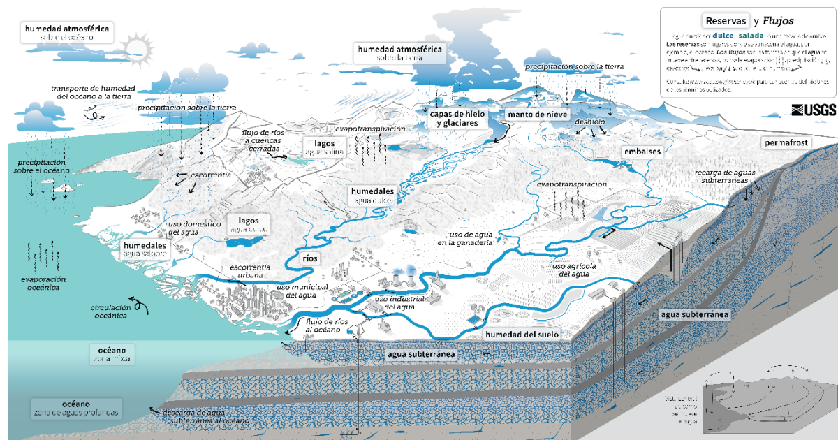
Figura 19. Esquema del ciclo hidrológico. Fuente: United States Geological Survey
