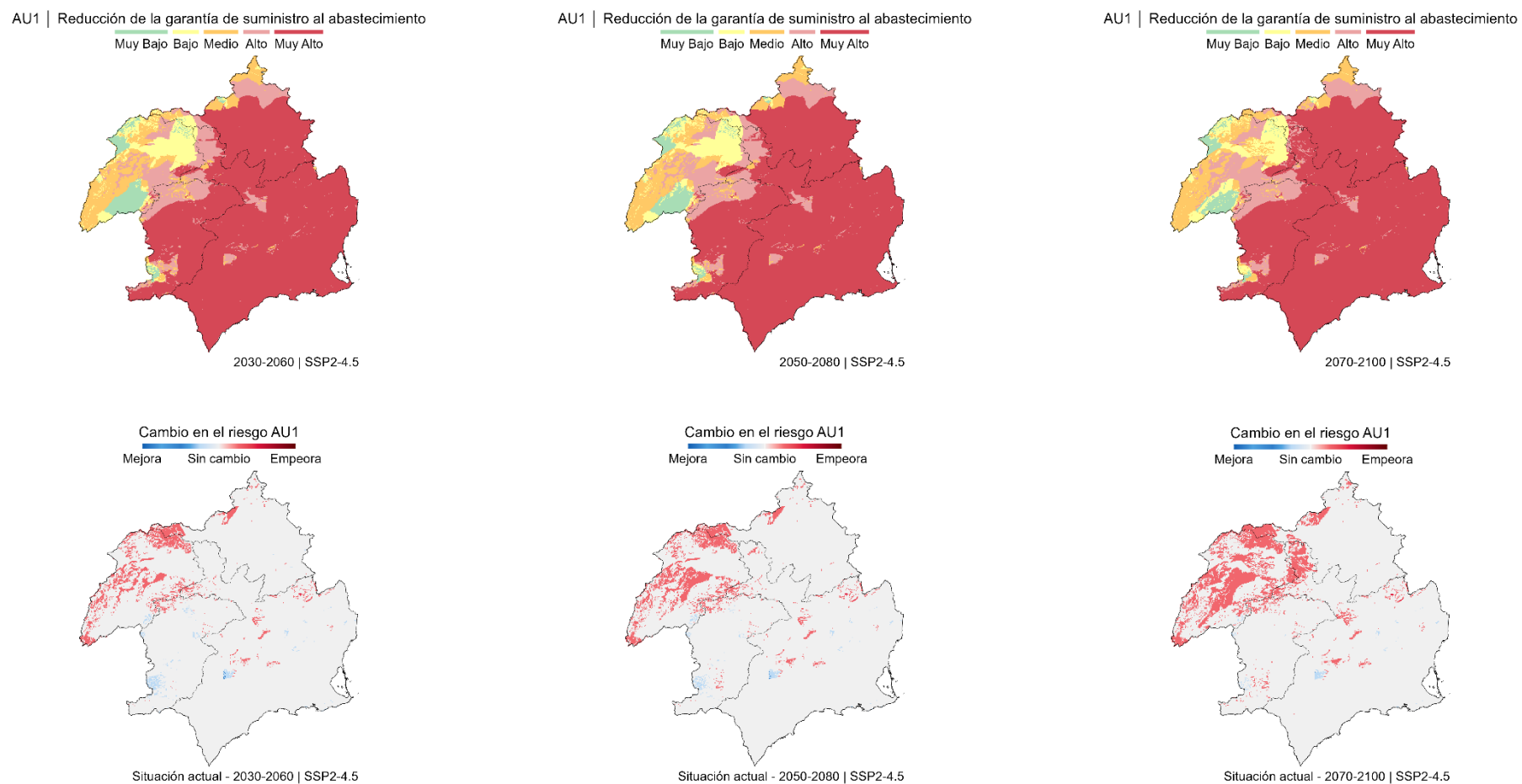
Figura 122. Evaluación del riesgo AU1 proyectado bajo el escenario intermedio (SSP2-4.5), para los horizontes temporales 2030-2060, 2050-2080 y 2070-2100 respecto a la situación de riesgo actual.
