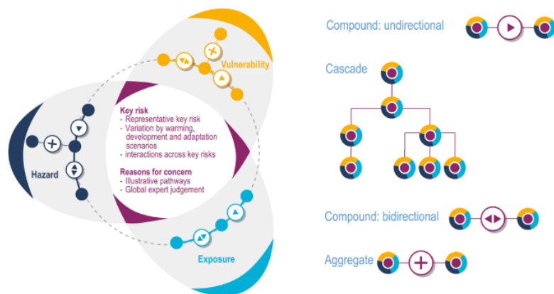
Figura 69. Marco conceptual del riesgo en el AR6. (IPCC WGII AR6, 2022).
