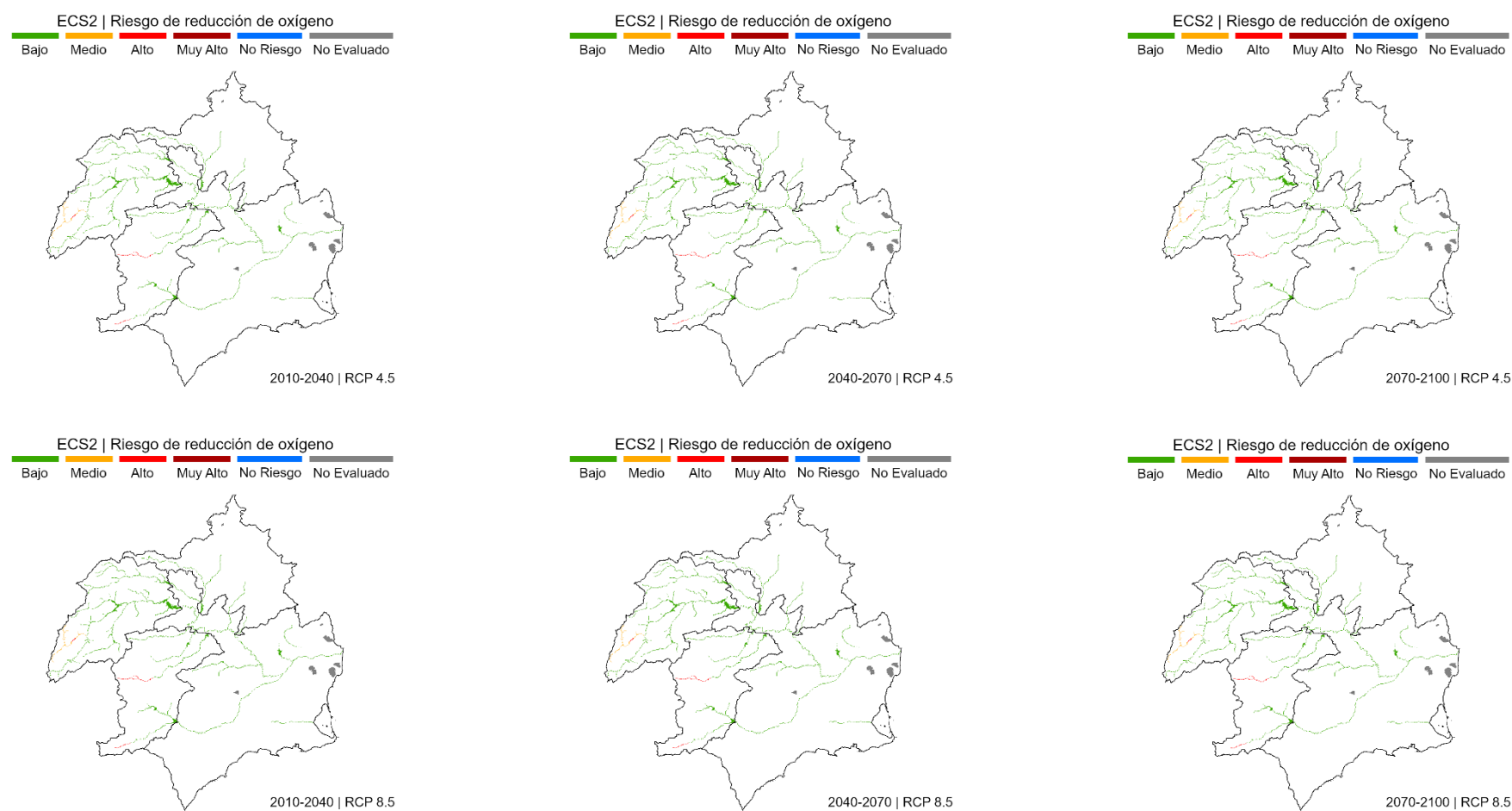
Figura 95. Evaluación del riesgo ECS2 proyectado bajo los escenarios RCP 4.5 y RCP 8.5, para los horizontes temporales 2010-2040, 2040-2070 y 2070-2100. Riesgo de reducción de oxígeno.
