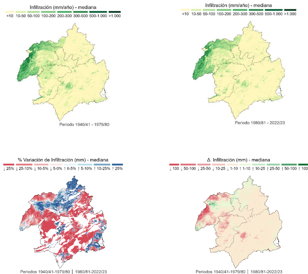
Figura 27. Caracterización espacial y temporal de la infiltración. Comparación entre los periodos 1940/41–1979/80 y 1980/81–2022/23. Fuente: Elaboración propia a partir de información de SIMPA (CEDEX).
