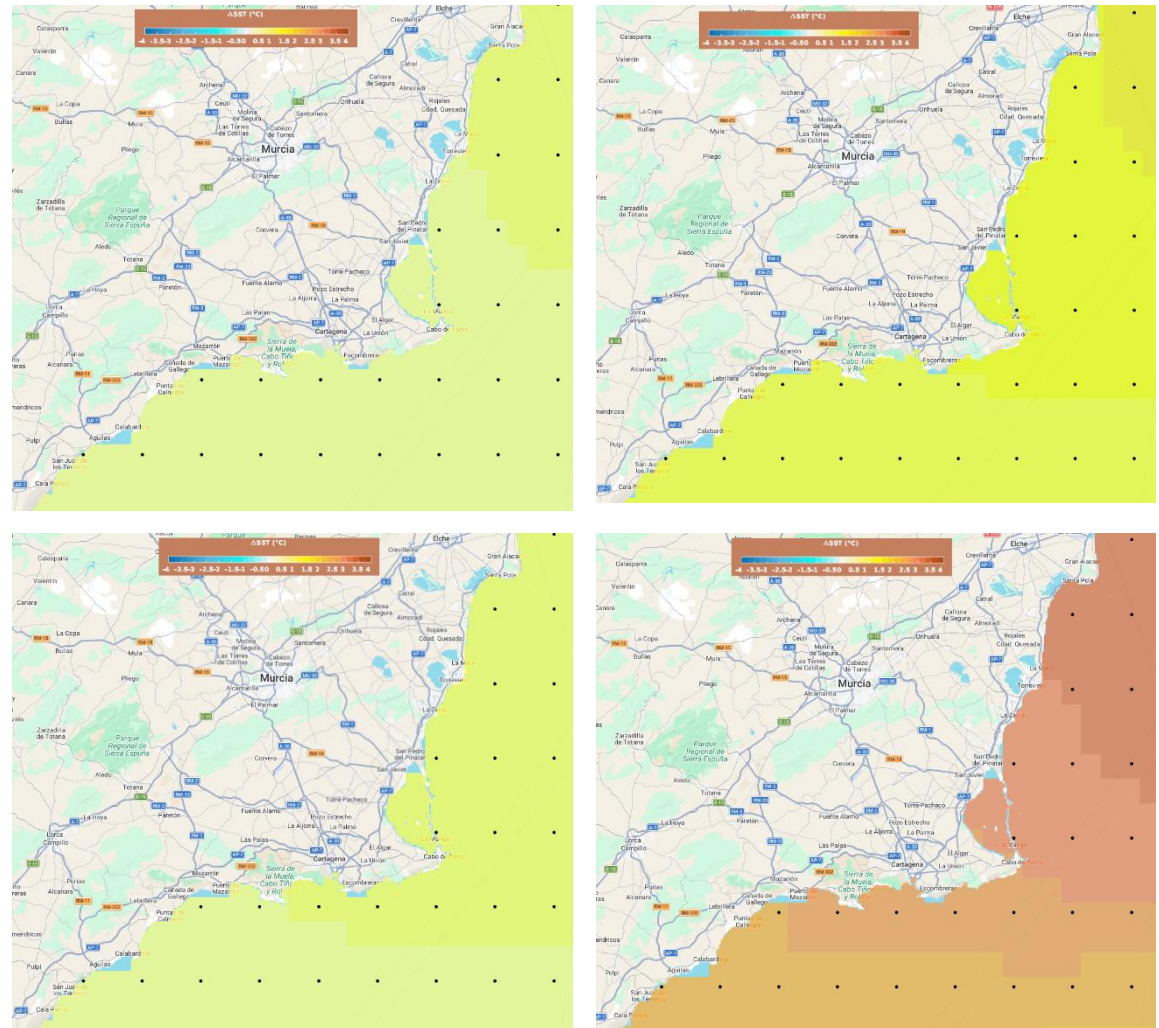
Figura 67. Variación de la temperatura media de la superficie del mar bajo los escenarios RCP-4.5 (arriba) y RCP 8.5 (debajo). Fuente: IH Cantabria
