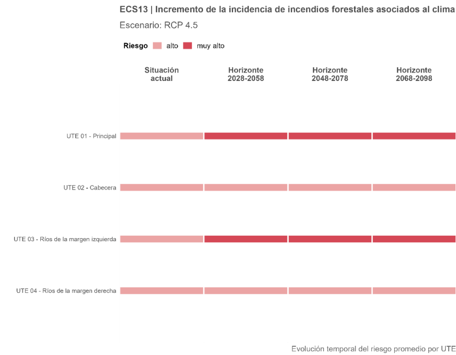
Figura 118. Trayectoria temporal del riesgo ECS13 promedio por UTE, proyectado bajo el escenario intermedio (SSP2-4.5).
