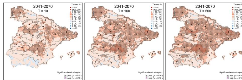
Figura 44. Tasas de cambio en cuantil medias para precipitación diaria máxima anual; modelo GEV-L en RCP 8.5. Fuente: CEDEX
