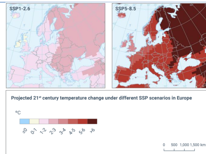
Figura 40. Tendencia en la temperatura media anual en Europa bajo diferentes escenarios climáticos. Fuente: AEMA
