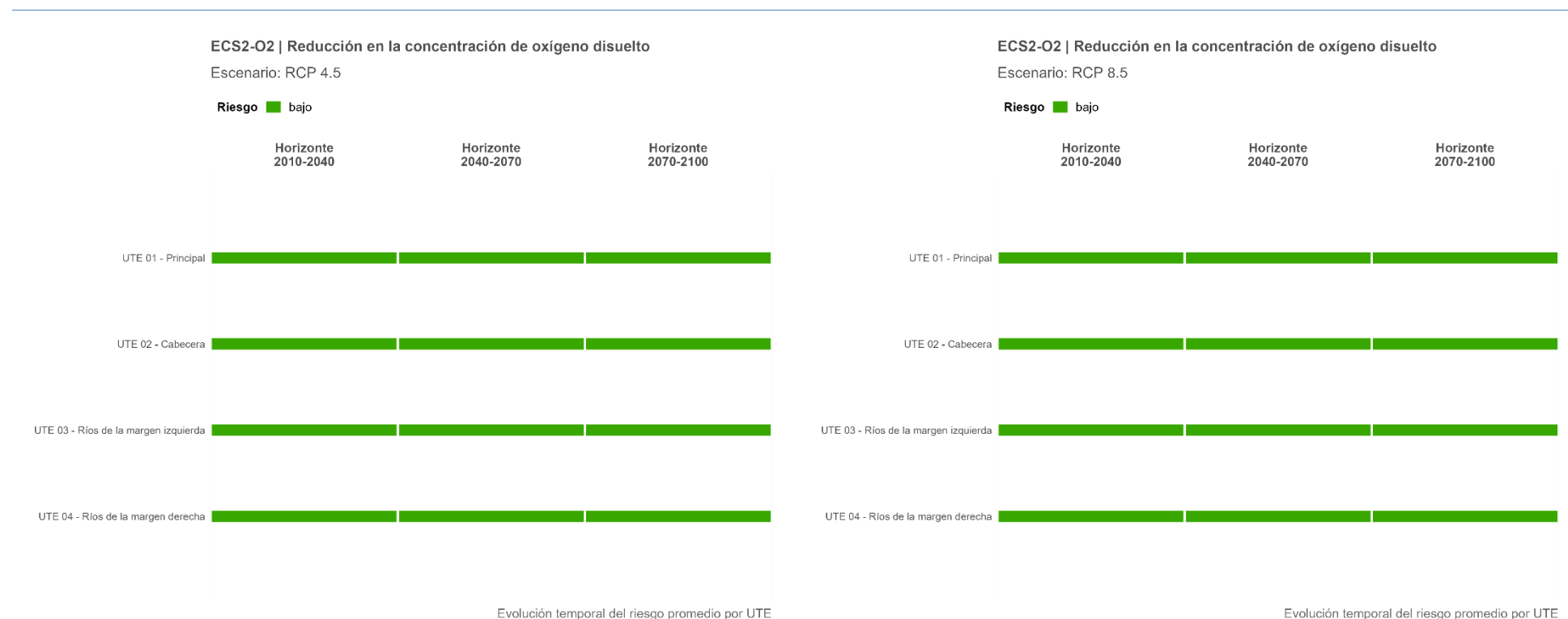
Figura 99. Trayectoria temporal del riesgo ECS2-O2 promedio por UTE, proyectado bajo el escenario intermedio (RCP 4.5)
