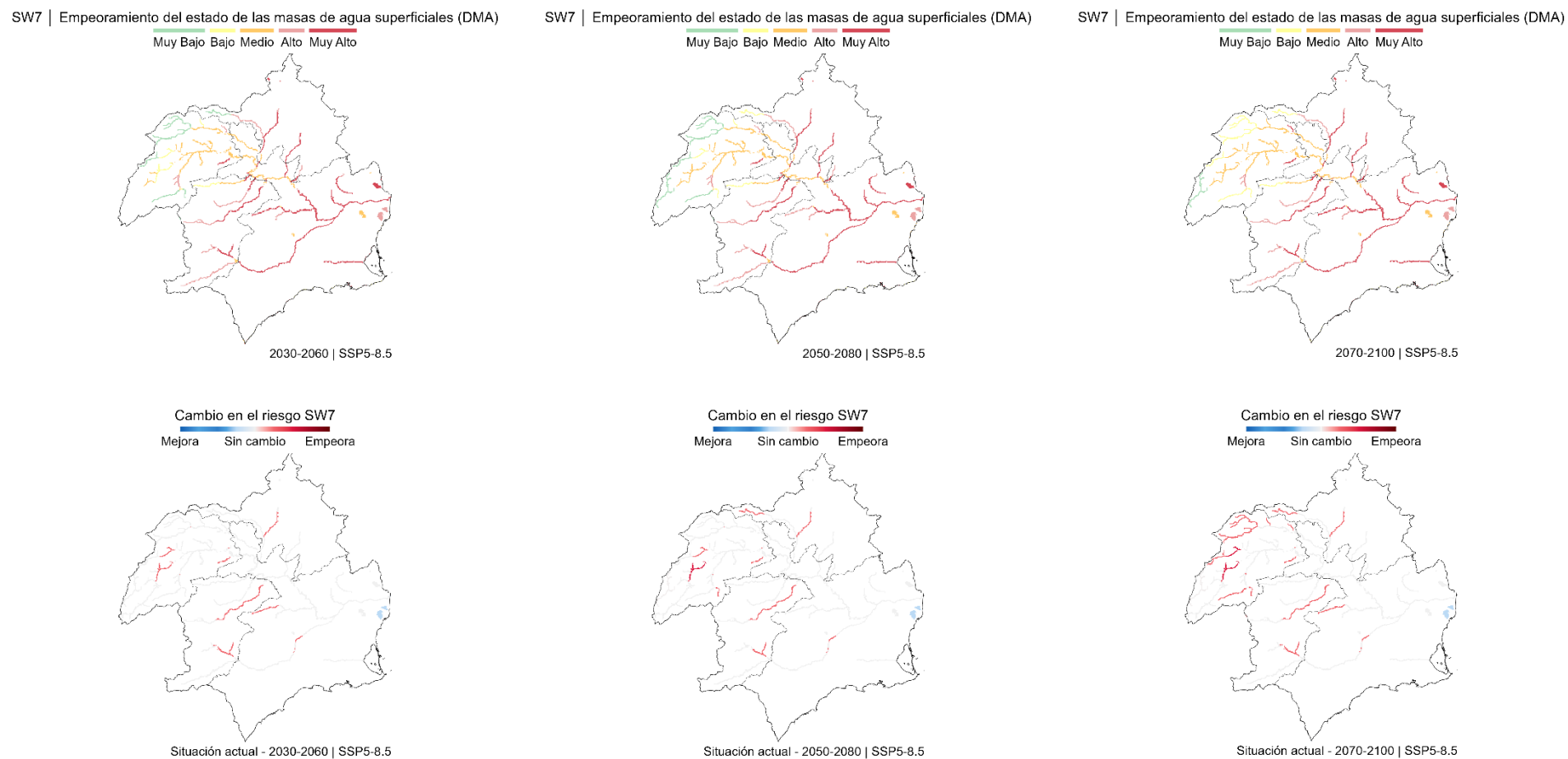
Figura 84. Evaluación del riesgo SW7 proyectado bajo el escenario de altas emisiones (SSP5-8.5), para los horizontes temporales 2030-2060, 2050-2080 y 2070-2100 respecto a la situación de riesgo actual.
