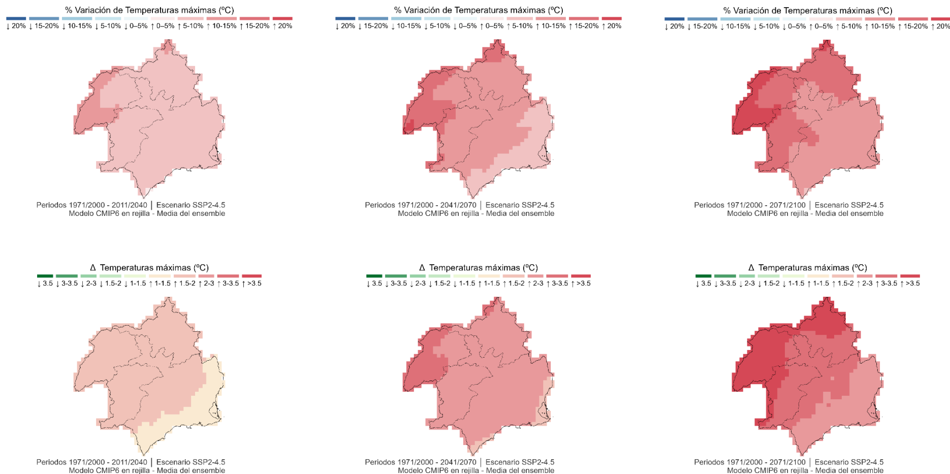
Figura 46. Variación de las temperaturas máximas proyectadas bajo el escenario intermedio de emisiones (SSP2-4.5), para los horizontes temporales 2011-2040, 2041-2070 y 2071-2100, en comparación con el periodo de control 1971-2000. Fuente: Elaboración propia a partir de información de AdapteCCA.
