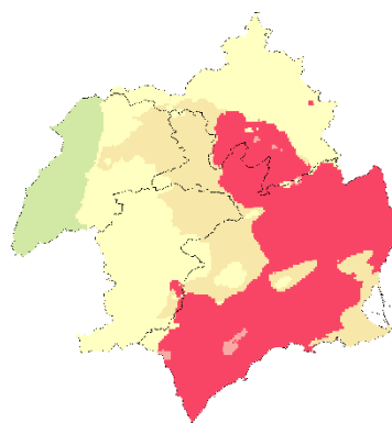
Figura 45. Variación de tipos climáticos bajo los escenarios intermedio (SSP2-4.5) y de altas emisiones (SSP5-8.5) para los horizontes temporales 2011-2040, 2041-2070 y 2071-2100. Fuente: AEMET
