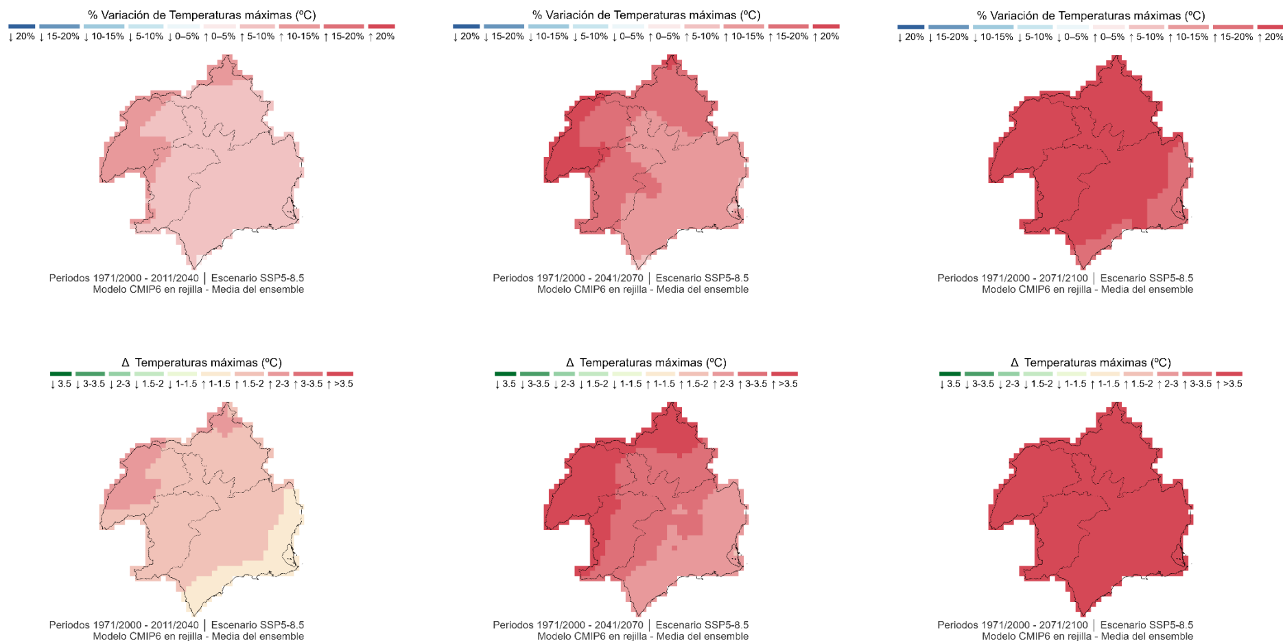
Figura 47. Variación de las temperaturas máximas proyectadas bajo el escenario pesimista de emisiones (SSP5-8.5), para los horizontes temporales 2011-2040, 2041-2070 y 2071-2100, en comparación con el periodo de control 1971-2000. Fuente: Elaboración propia a partir de información de AdapteCCA.
