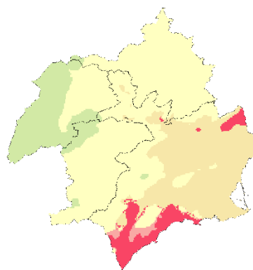
Figura 45. Variación de tipos climáticos bajo los escenarios intermedio (SSP2-4.5) y de altas emisiones (SSP5-8.5) para los horizontes temporales 2011-2040, 2041-2070 y 2071-2100. Fuente: AEMET
