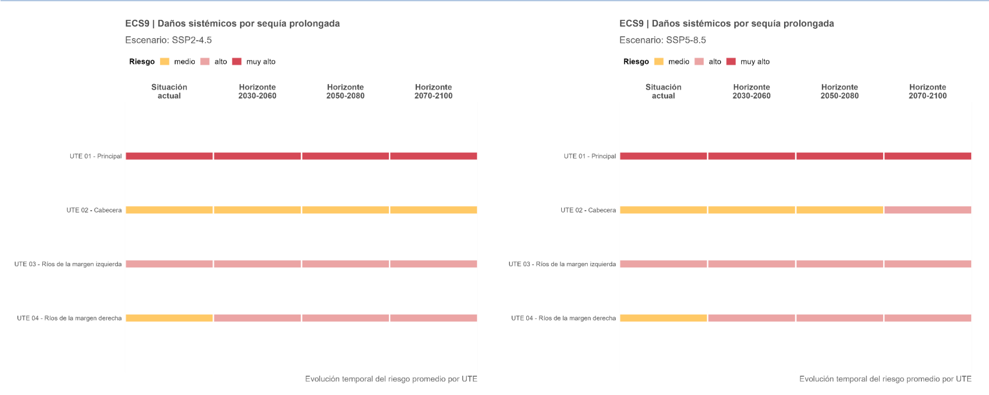
Figura 109. Trayectoria temporal del riesgo ECS9 promedio por UTE, proyectado bajo el escenario intermedio (SSP2-4.5).
