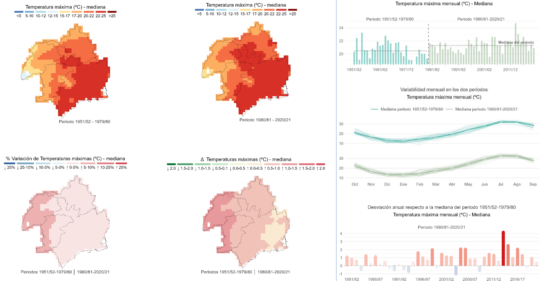
Figura 22. Caracterización espacial y temporal de la temperatura máxima. Comparación entre los periodos 1951/52-1979/80 y 1980/81-2020/21. Fuente: Elaboración propia a partir de información de Adapteca.
