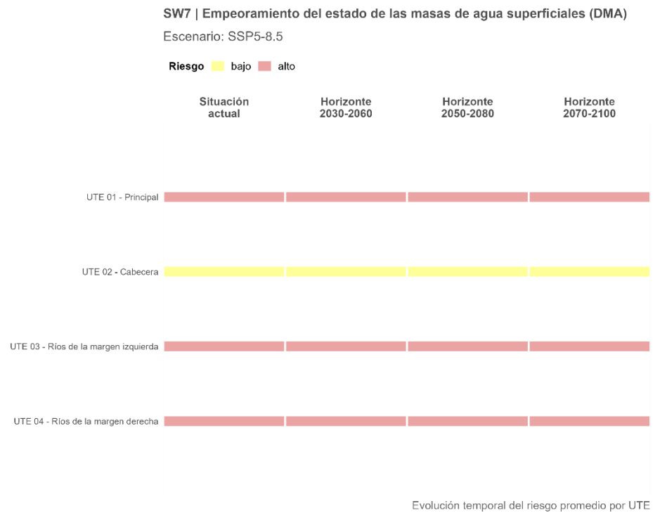
Figura 86. Trayectoria temporal del riesgo SW7 promedio por UTE, proyectado bajo el escenario de altas emisiones (SSP5-8.5).
