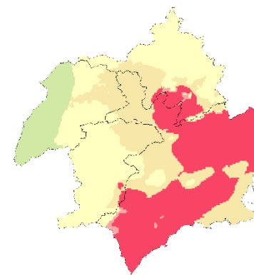
Clasificación climática de Köppen-Geiger (2071-2100) | Escenario SSP5-8.5
