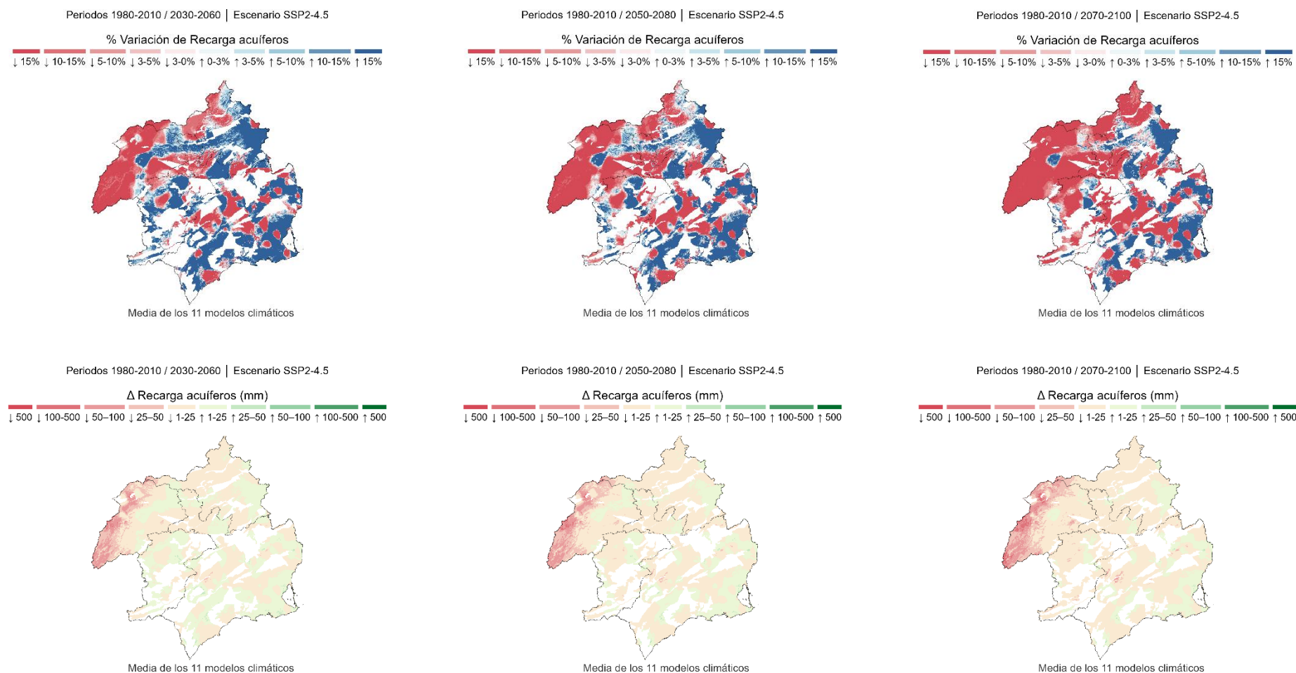
Figura 52. Variación de la infiltración proyectada bajo el escenario intermedio de emisiones (SSP2-4.5), para los horizontes temporales 2030-2060, 2050-2080 Y 2070-2100, en comparación con el periodo de control 1980-2010. Fuente: Elaboración propia a partir de información del CEDEX, 2025.
