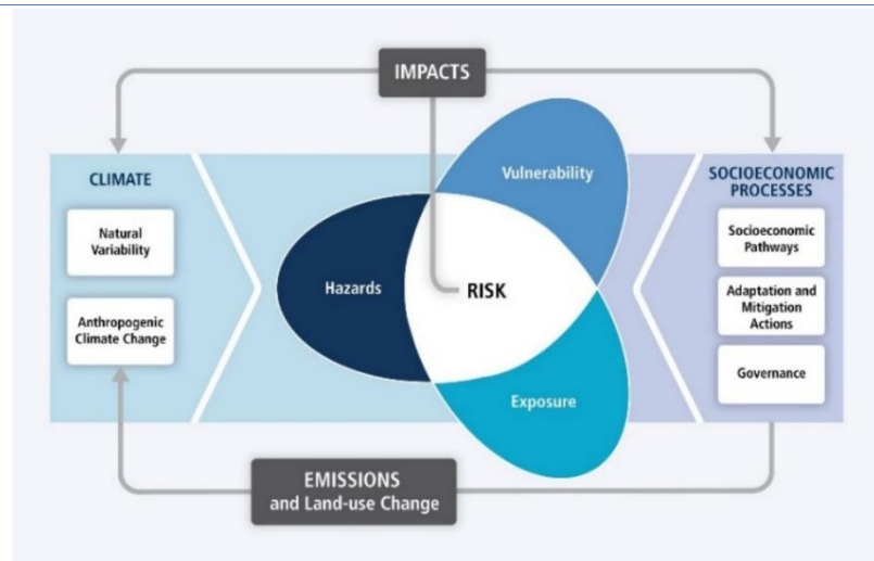
Figura 68. Marco conceptual para la evaluación del riesgo. (IPCC WGII AR5, 2014).
