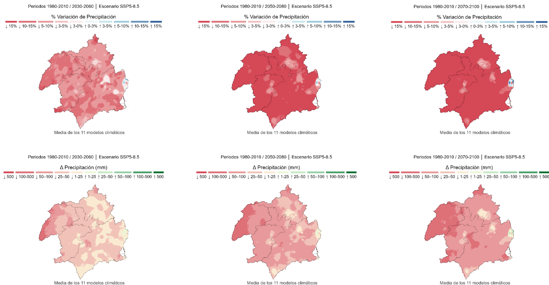
Figura 49. Variación de la precipitación proyectada bajo el escenario de altas emisiones (SSP5-8.5), para los horizontes temporales 2030-2060, 2050-2080 Y 2070-2100, en comparación con el periodo de control 1980-2010. Fuente: Elaboración propia a partir de información del CEDEX, 2025.
