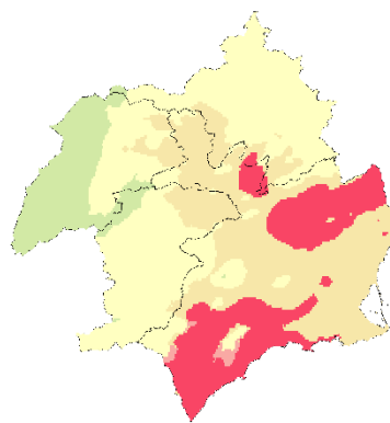
Clasificación climática de Köppen-Geiger (2041-2070) | Escenario SSP5-8.5
