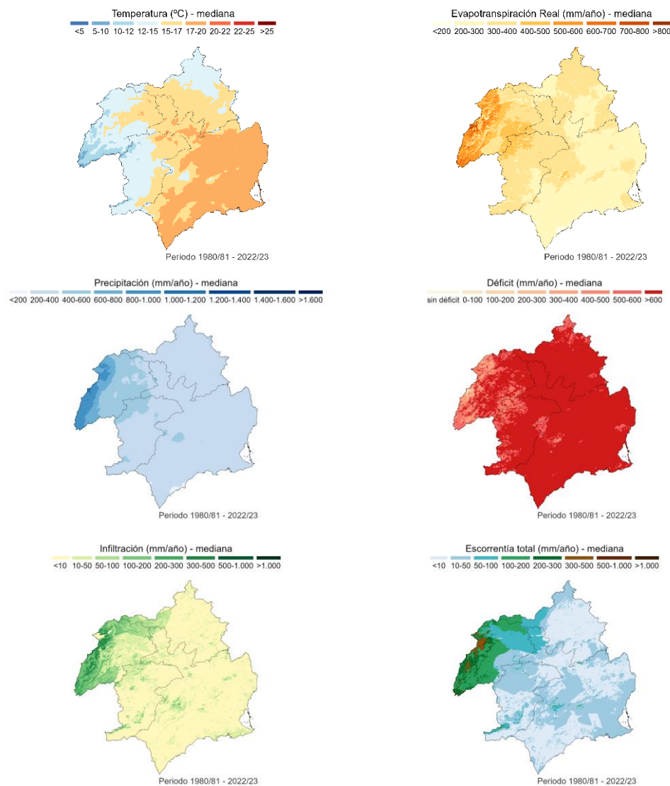
Figura 2. Variables atmosféricas e hidrológicas en el periodo 1980/81 – 2022/23. Fuente: SIMPA
