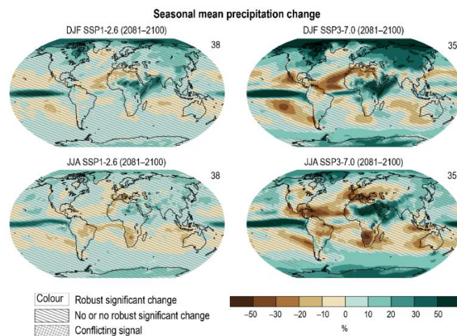
Figura 41. Cambio a largo plazo de la precipitación media estacional. Fuente AR6 . DJF:diciembre-enero-febrero; JJA: junio-julio-agosto
