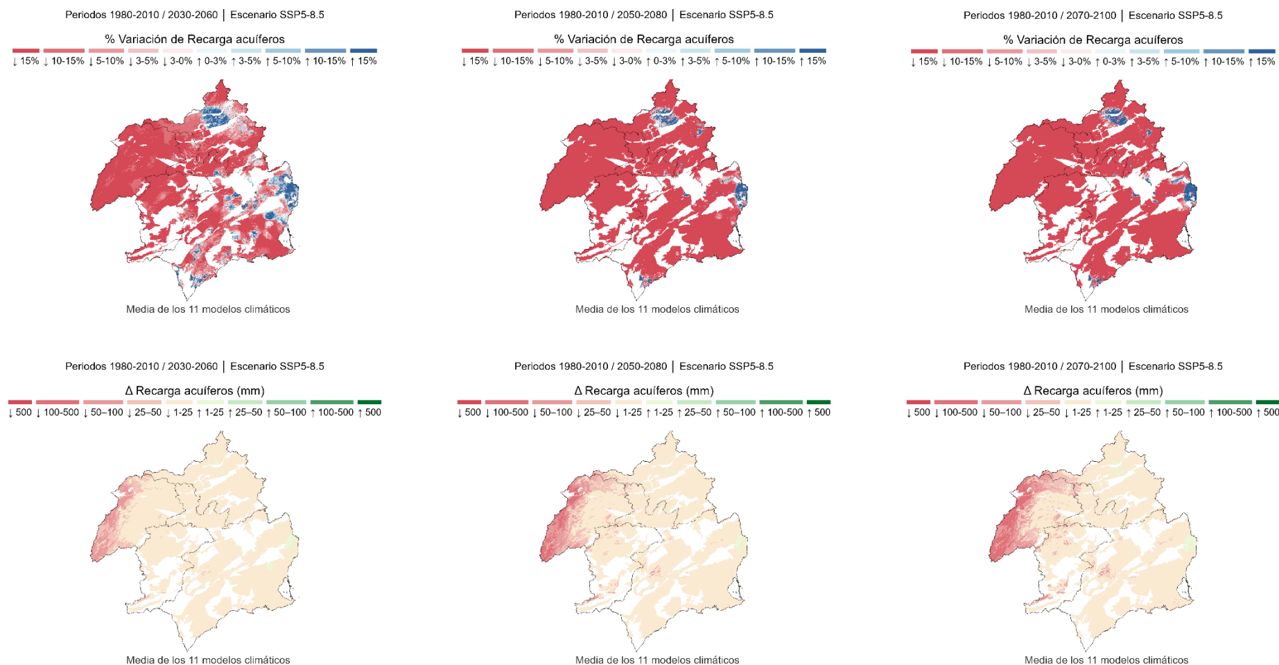
Figura 53. Variación de la infiltración proyectada bajo el escenario pesimista de emisiones (SSP5-8.5), para los horizontes temporales 2030-2060, 2050-2080 Y 2070-2100, en comparación con el periodo de control 1980-2010. Fuente: Elaboración propia a partir de información del CEDEX, 2025.
