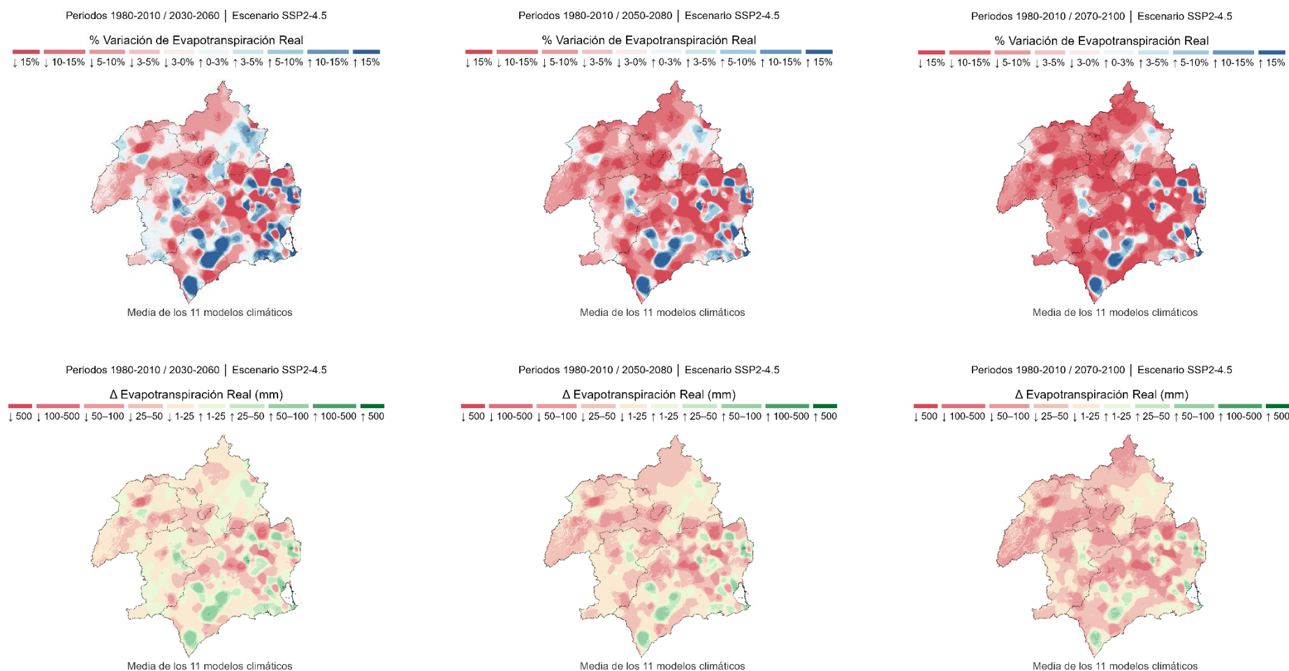
Figura 54. Variación de la evapotranspiración real proyectada bajo el escenario intermedio de emisiones (SSP2-4.5), para los horizontes temporales 2030-2060, 2050-2080 Y 2070-2100, en comparación con el periodo de control 1980-2010. Fuente: Elaboración propia a partir de información del CEDEX, 2025.
