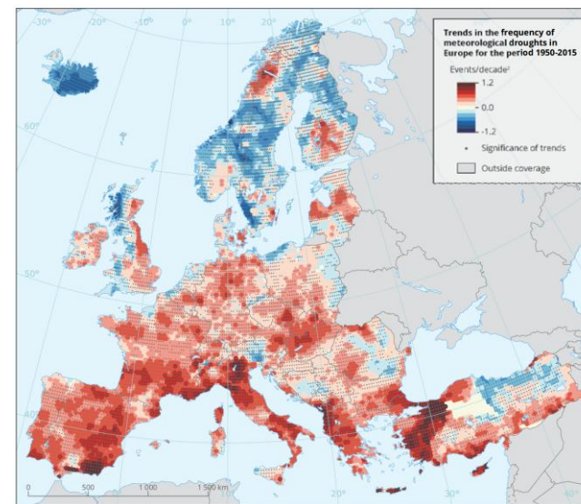
Figura 18. Tendencias en la frecuencia de sequías meteorológicas en Europa durante el período 1950–2015. Fuente: AEMA 2021 .
