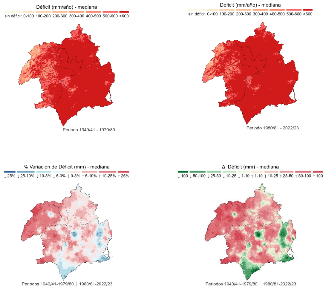
Figura 28. Caracterización espacial y temporal del déficit. Comparación entre los periodos 1940/41–1979/80 y 1980/81–2022/23. Fuente: Elaboración propia a partir de información de SIMPA (CEDEX).
