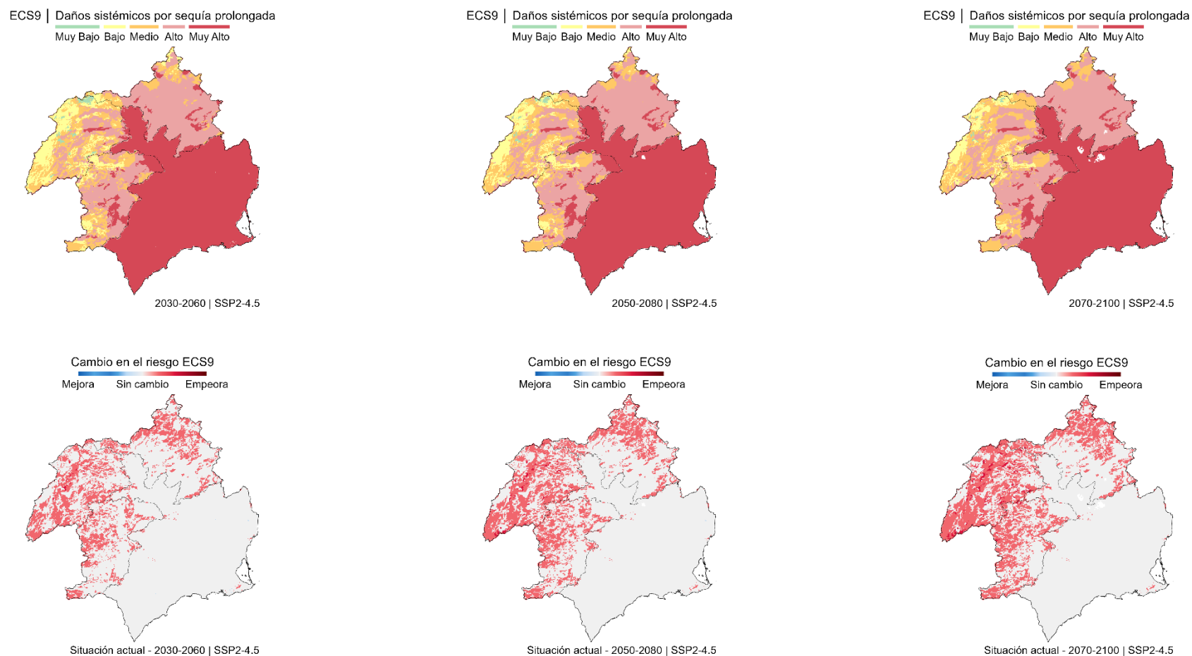
Figura 107. Evaluación del riesgo ECS9 proyectado bajo el escenario intermedio (SSP2-4.5), para los horizontes temporales 2030/2060, 2050/2080 y 2070/2100 respecto a la situación de riesgo actual.
