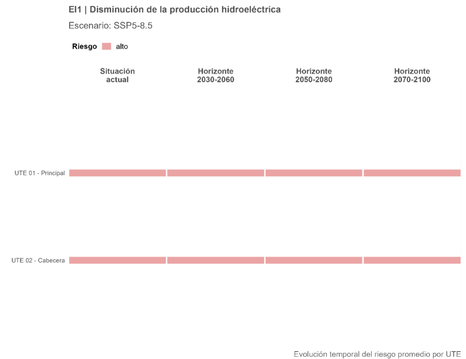
Figura 137. Trayectoria temporal del riesgo EI1 promedio por UTE, proyectado bajo el escenario de altas emisiones (SSP5-8.5).
