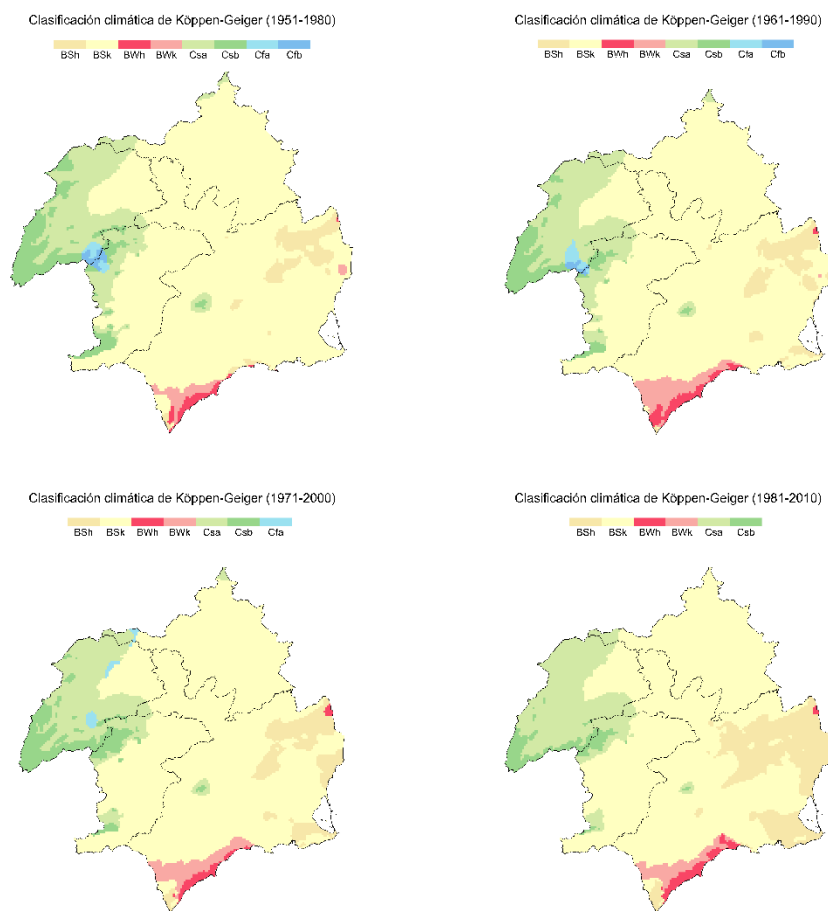
Figura 14. Tipos de clima y su evolución en el periodo 1950 y 2010
