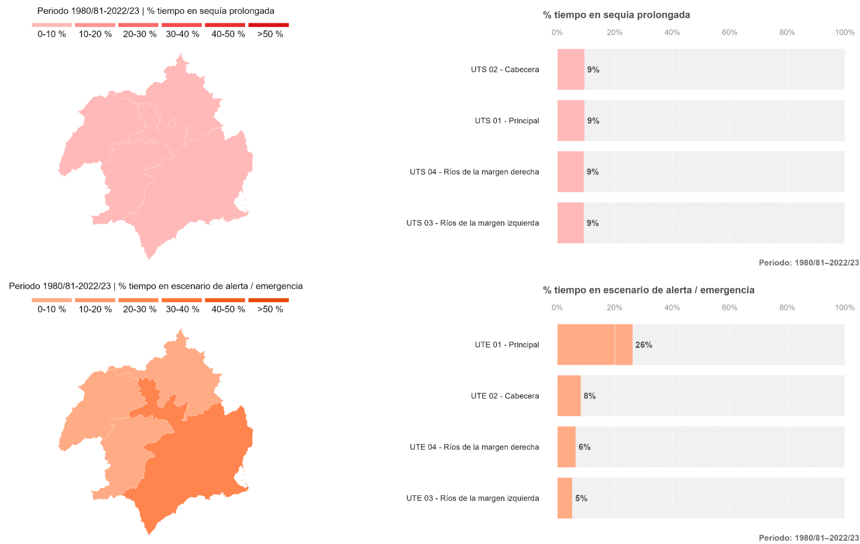
Figura 36. Caracterización espacial y temporal de la sequía prolongada y escasez coyuntural. Fuente: elaboración a partir de los informes mensuales de seguimiento de los PES. Todas las UTS cuentan con un porcentaje de tiempo en sequía prolongada del 9%. En cuanto a los escenarios de alerta o emergencia, la UTE con mayor porcentaje de tiempo en estas situaciones es la UTE 01 - Principal (26%) y la que registra el menor porcentaje es la UTE 03 - Ríos Margen izquierda (5%).
