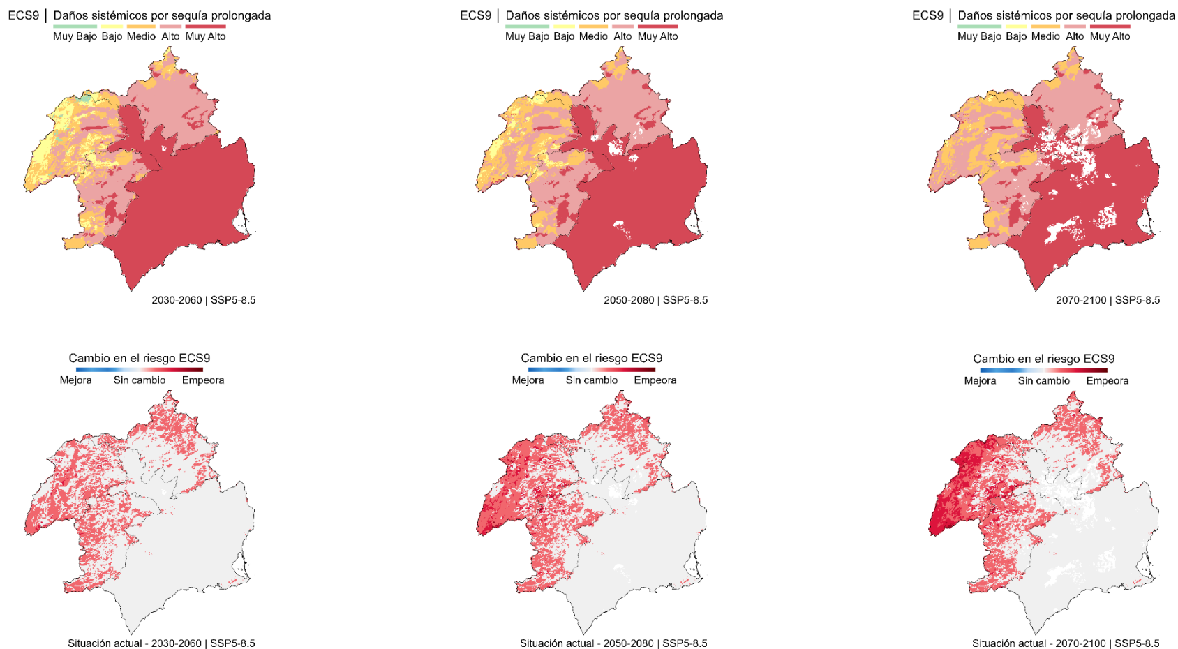
Figura 108. Evaluación del riesgo ECS9 proyectado bajo el escenario de altas emisiones (SSP5-8.5), para los horizontes temporales 2030/2060, 2050/2080 y 2070/2100 respecto a la situación de riesgo actual.
