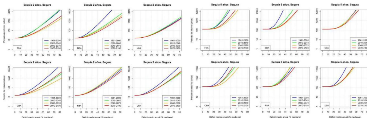
Figura 64. Periodo de retorno de sequías en España para diferentes déficits medios anuales y duración 2 años (izquierda) y 5 años (derecha) para el periodo de control (1961-200) y tres periodos futuros (2010-2040, 2040-2070 y 2070-2100) con el escenario climático de altas emisiones (RCP 8.5)
