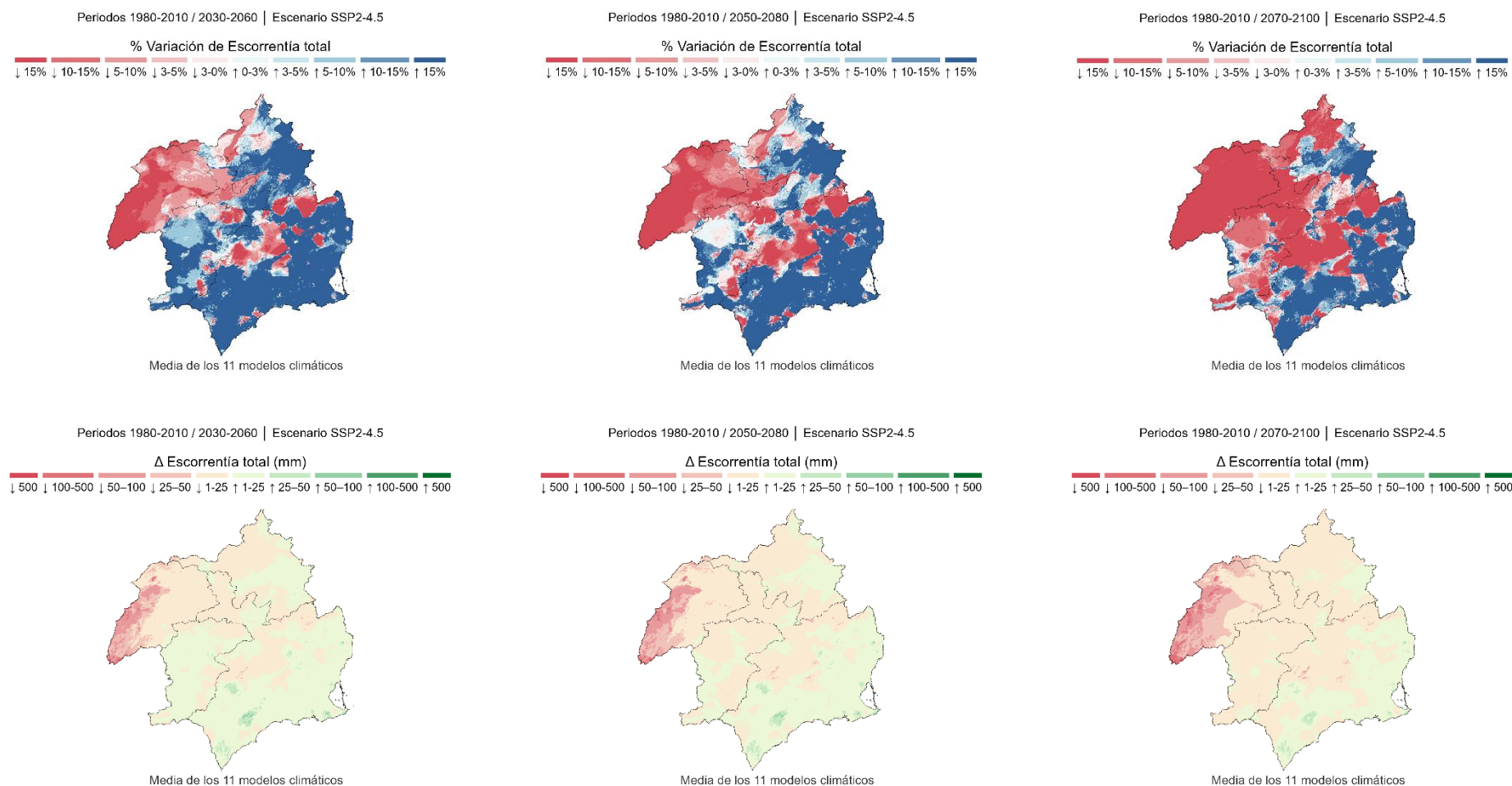
Figura 56. Variación de las aportaciones totales proyectadas bajo el escenario intermedio de emisiones (SSP2-4.5), para los horizontes temporales 2030-2060, 2050-2080 Y 2070-2100, en comparación con el periodo de control 1980-2010. Fuente: Elaboración propia a partir de información del CEDEX, 2025.
