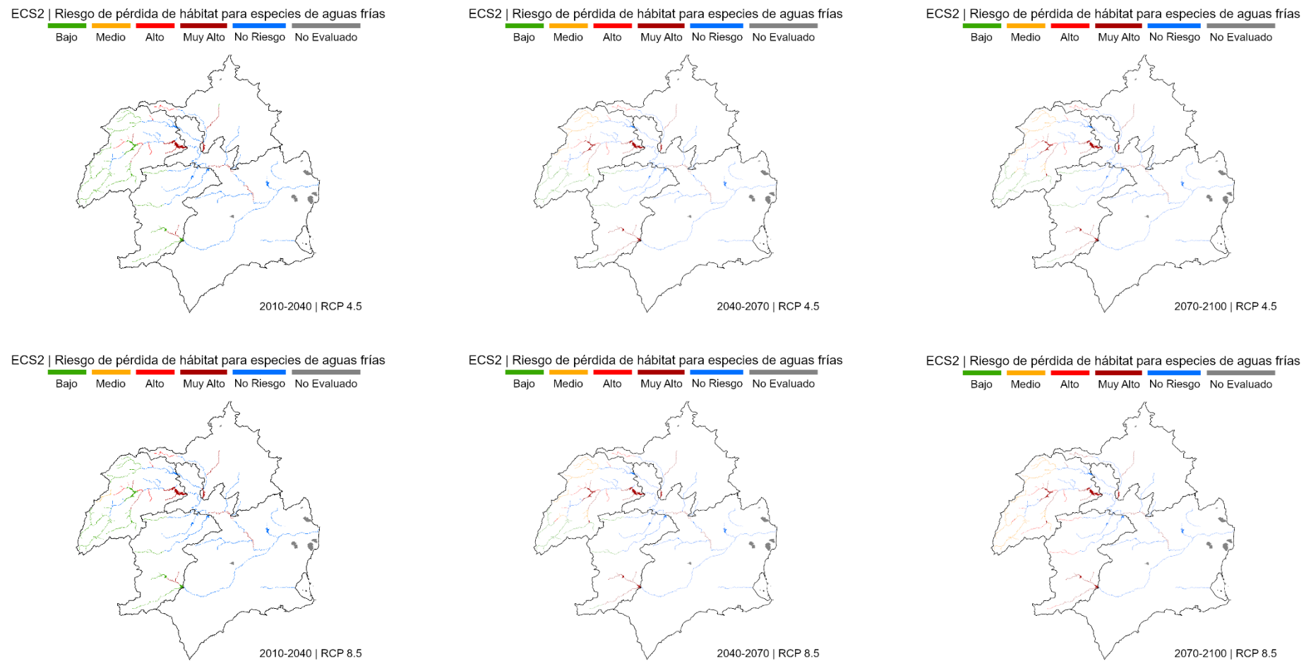
Figura 94. Evaluación del riesgo ECS2 proyectado bajo los escenarios RCP 4.5 y RCP 8.5, para los horizontes temporales 2010-2040, 2040-2070 y 2070-2100. Riesgo de pérdida de hábitat para especies de aguas frías.
