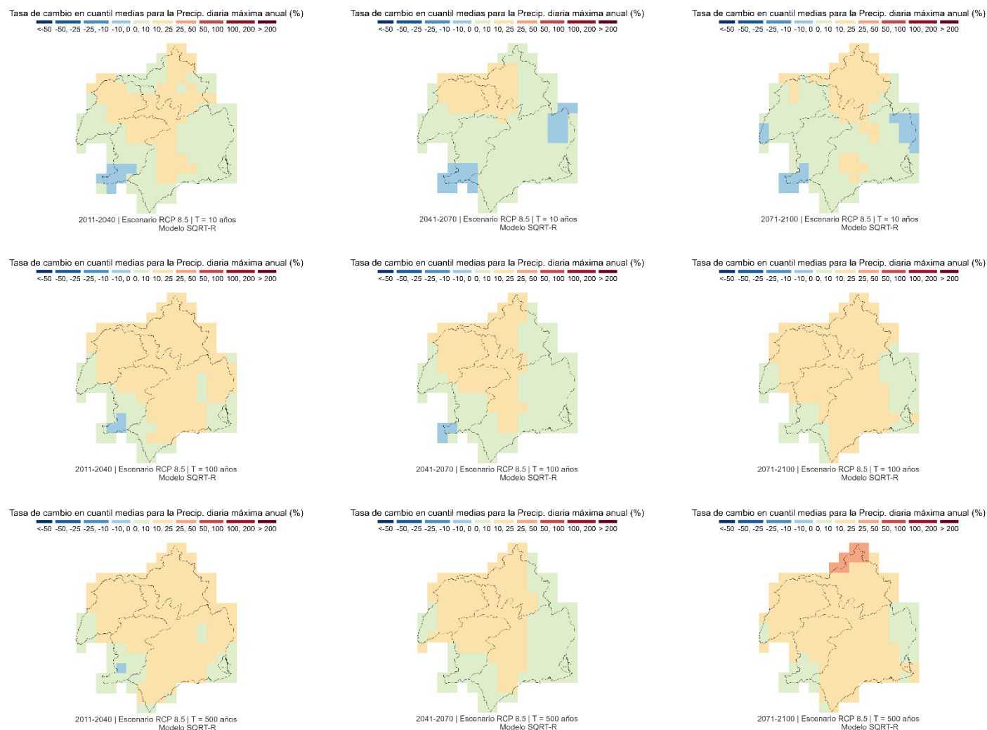
Figura 59. Tasa de cambio de la precipitación diaria máxima anual proyectada bajo el escenario de altas emisiones (SSP5-8.5) (RCP 8.5) para los horizontes temporales 2011-2040, 2041-2070 y 2071-2100, y para los periodos de retorno de 10, 100 y 500 años, calculada respecto al periodo de control (1971-2000). Fuente: elaboración propia a partir de información del CEDEX
