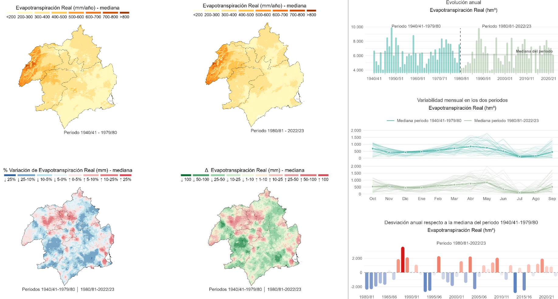
Figura 29. Caracterización espacial y temporal de la evapotranspiración real. Comparación entre los periodos 1940/41–1979/80 y 1980/81–2022/23. Fuente: Elaboración propia a partir de información de SIMPA (CEDEX).
