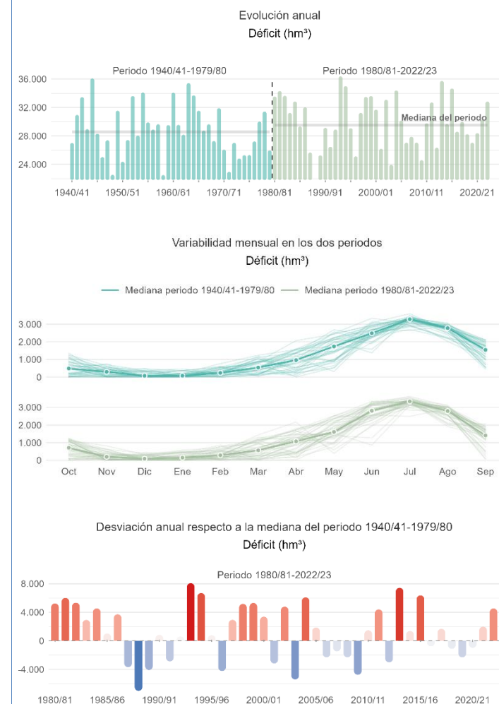
Figura 28. Caracterización espacial y temporal del déficit. Comparación entre los periodos 1940/41–1979/80 y 1980/81–2022/23. Fuente: Elaboración propia a partir de información de SIMPA (CEDEX).
