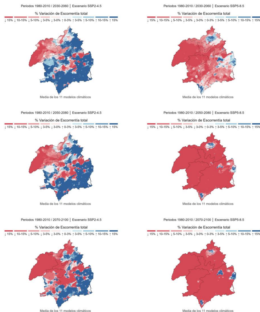
Figura 3. Evolución de la escorrentía total bajo los escenarios y horizontes de análisis
