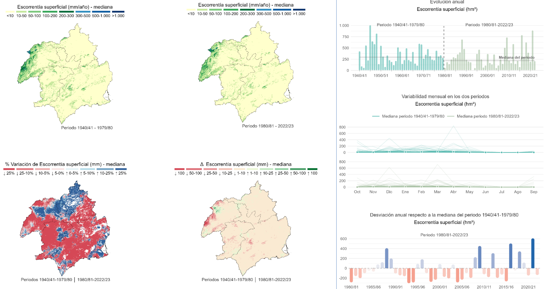
Figura 31. Caracterización espacial y temporal de la escorrentía superficial. Comparación entre los periodos 1940/41–1979/80 y 1980/81–2022/23. Fuente: Elaboración propia a partir de información de SIMPA (CEDEX).
