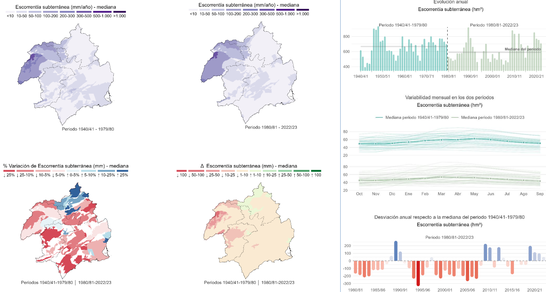
Figura 30. Caracterización espacial y temporal de la escorrentía subterránea. Comparación entre los periodos 1940/41–1979/80 y 1980/81–2022/23. Fuente: Elaboración propia a partir de información de SIMPA (CEDEX).
