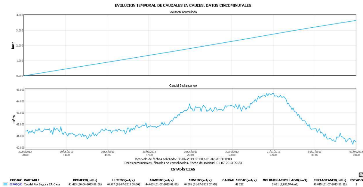
Variación del caudal registrado en la estación de alerta de Cieza durante el transcurso del episodio.
