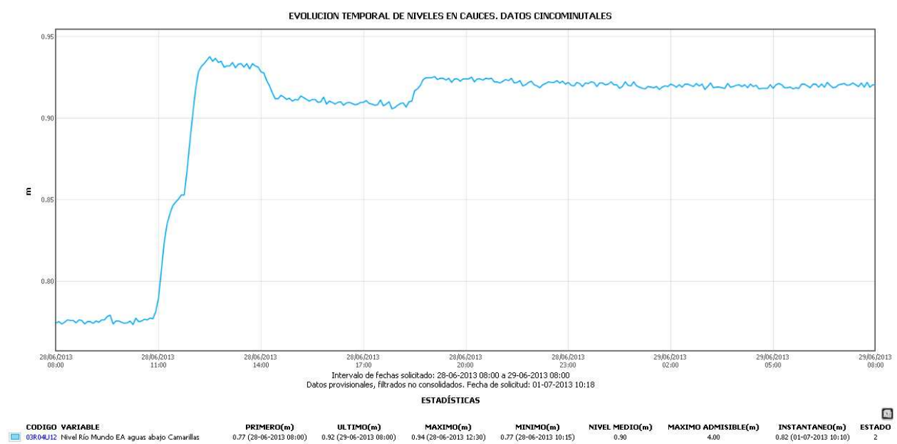
Variación del nivel registrado aguas abajo del embalse de Camarillas durante el transcurso del episodio.
