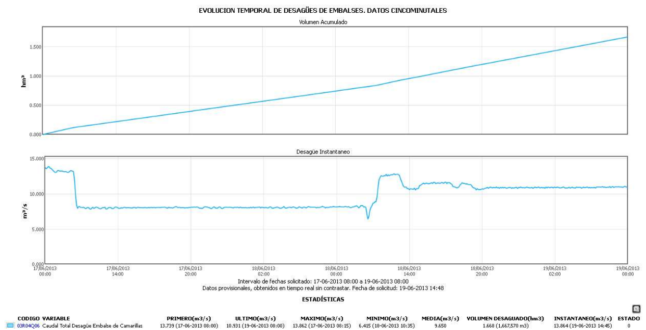
Variación del caudal de desagüe registrado en el embalse de Camarillas durante el transcurso del episodio.
