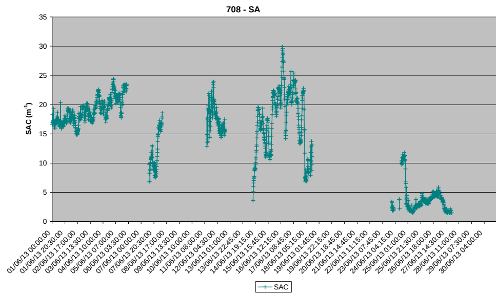
Valores del SAC registrados en la estación de alerta de San Antón durante el mes de Junio.
