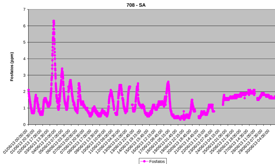
Concentración de fosfatos registrados en la estación de alerta de San Antón durante el mes de Junio.
