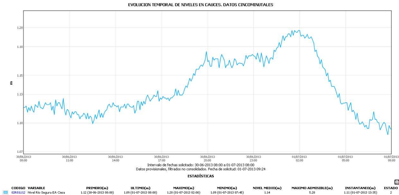
Variación del nivel registrado en la estación de alerta de Cieza durante el transcurso del episodio.
